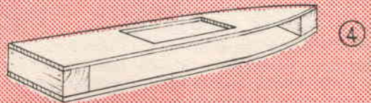
N. 4 - La imbarcazione composta del fondo, della coperta e dei due blocchi spaziatori, in queste condizioni, stanno per essere applicate le fiancate
