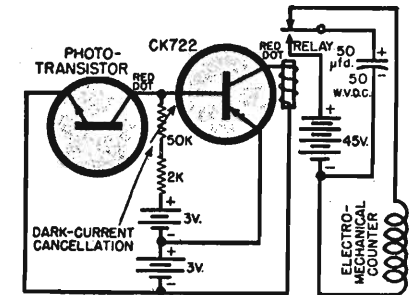
Fig. 2. - Circuito più complesso, che comprende uno stadio amplificatore e che consente una sensibilità da 3 a 6 volte maggiore.
