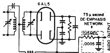
Fig. 2. - Il circuito « ratio-detector » richiede lo stesso circuito di de-emfasi. Nel testo è ampiamente spiegato come si debba procedere al calcolo della costante di tempo.
