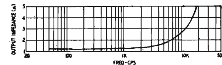
Fig. 5. - L'impedenza d'uscita è inferiore ai 2 ohm fino a 7.000 Hz.
