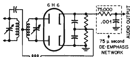
Fig. 1. - Questo è un classico circuito discriminatore nel quale il circuito di de-emfasi, costituito da una resistenza e da una capacità, può venire facilmente identificato, controllato e corretto.
