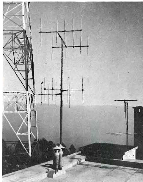
Un particolare del centro trasmettente di Portofino che sorge sull'omonimo promontorio alla quota di 420 m.
