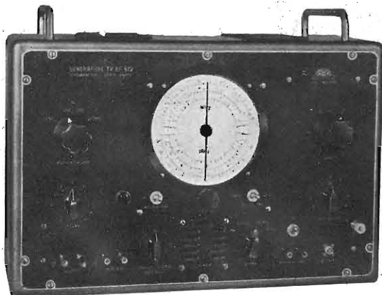
Il Generatore TV EP812 della UNA, illustrato qui accanto, comprende un Calibratore ed un Generatore di barre. Si tratta di un complesso preciso e compatto, indispensabile per il servizio TV.
