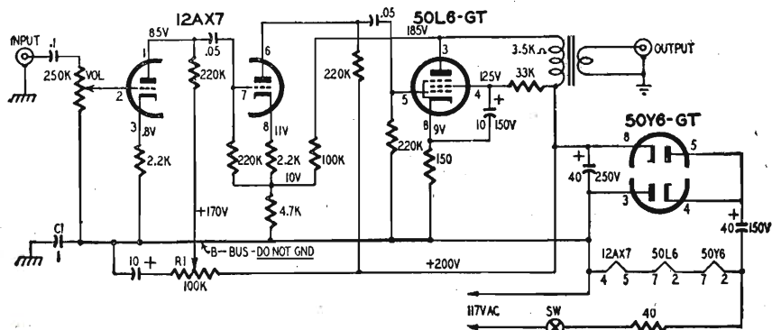
Fig. 1. - Il circuito elettrico. Come per ogni apparecchio senza trasformatore di alimentazione, il negativo e la massa devono essere distinti e uniti solo dal condensatore C1.
