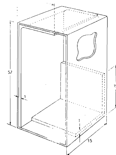
Fig. 5. - Nell'interno della custodia « R. J. » viene eseguito un rivestimento di materiale assorbente nelle posizioni indicate in figura.
