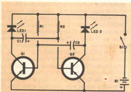
Fig. 3 - I LED lampeggiatori possono essere usati in una grande varietà di giocattoli.
