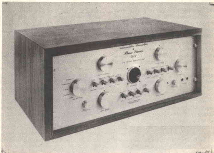
Questo preamplificatore a quattro canali della Phase Linear, denominato "Autocorrelation Preamplifier", è dotato di speciali circuiti per la riduzione del soffio e del rumore, di un rigeneratore della dinamica e di un equalizzatore attivo.
