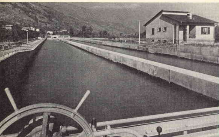
Canale derivatore all'aperto annesso all'impianto SIP di Quart. La vasca di carico in questo caso svolge pure la funzione di volano idraulico.
