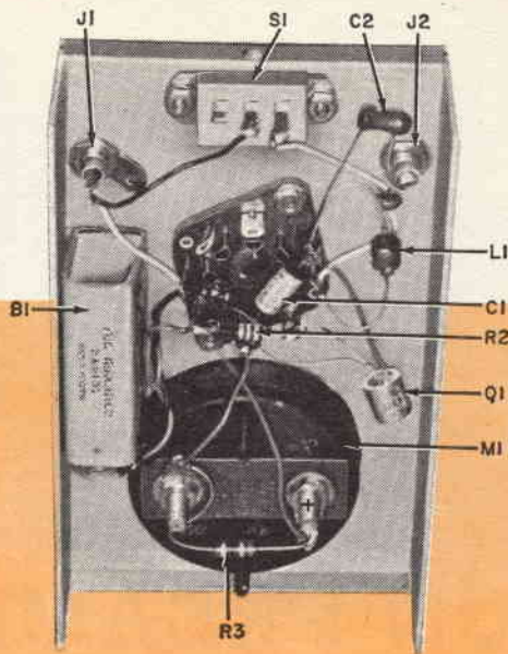
La disposizione dei componenti non è critica, tuttavia è consigliabile seguire la disposizione illustrata nella fotografia e nel disegno. I terminali inutilizzati sullo zoccolo portavalvole sono usati come linguette di ancoraggio isolate.
