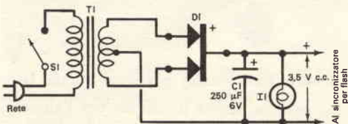
Schema elettrico del dispositivo. La lampada II scarica il condensatore quando si apre SI .
