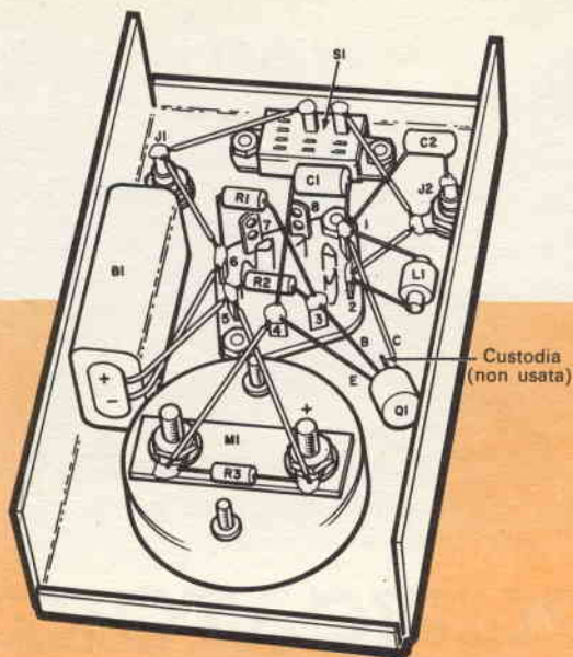
La disposizione dei componenti non è critica, tuttavia è consigliabile seguire la disposizione illustrata nella fotografia e nel disegno. I terminali inutilizzati sullo zoccolo portavalvole sono usati come linguette di ancoraggio isolate.
