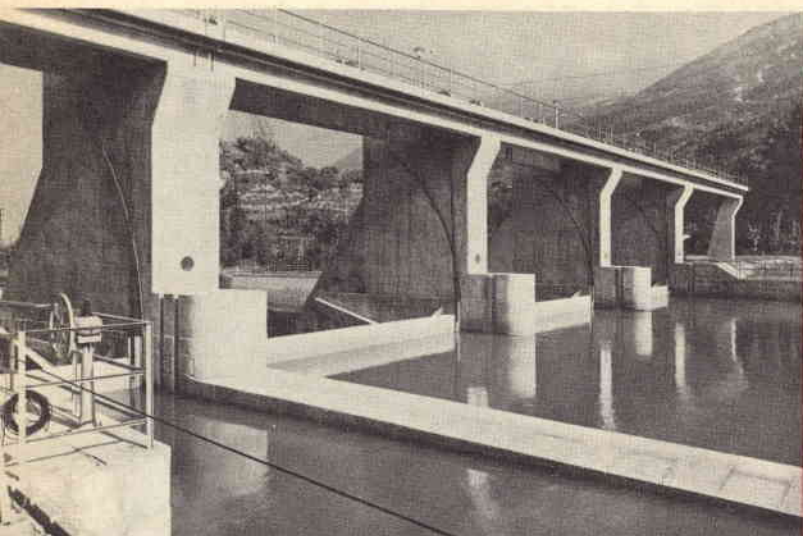
Nell'impianto SIP di Quart lo sbarramento della Dora è fatto con traverse in muratura.
