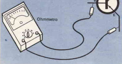
Fig. 2 - Un comune ohmmetro può essere impiegato per individuare cortocircuiti od interruzioni nelle giunzioni di un transistor.
