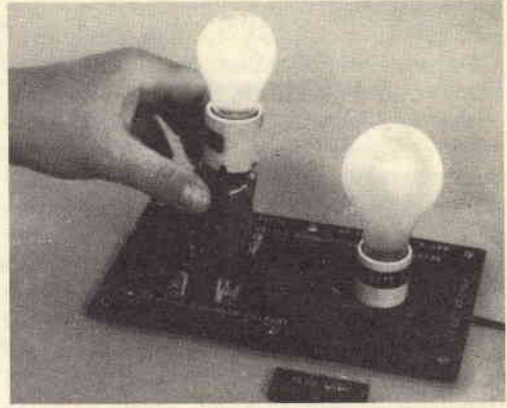
Fig. 3 - Il principio del trasformatore si può dimostrare facilmente sistemando l'insieme di L2/I2 su L1. In L2 viene indotta una tensione sufficiente a far brillare la lampada da 15 W (I2).
