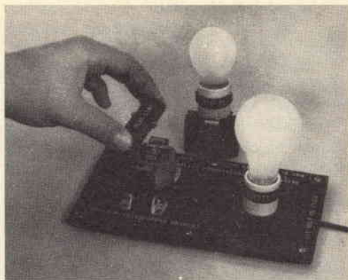
Fig. 1 - L'operatore toglie il giogo a forma di I dall'induttanza L1, riducendo l'induttanza della bobina e facendo di conseguenza brillare vivamente la lampada da 60 W (I1) collegata in serie.
