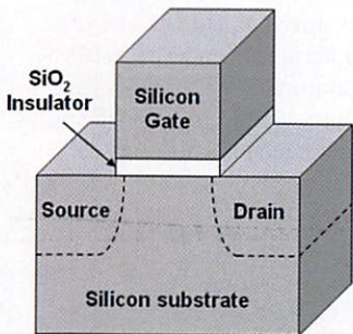
Transistor : l'Ancien (SiO 2 ) et le Nouveau (HK+Metal).
