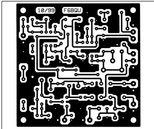
Circuit imprimé du TRX.
