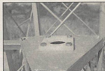
Détail de la cage avec pièce Rilsan.
