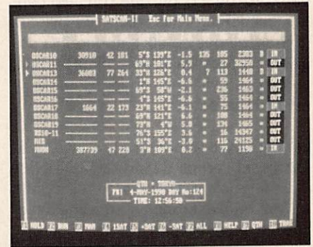
Position instantanée des satellites sélectionnés (vus de Tokyo dans cet exemple).
