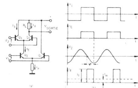
Fig. 5. - a) Discriminateur à coïncidence demi-onde simple. b) Formes d'ondes sur ce type de discriminateur.
