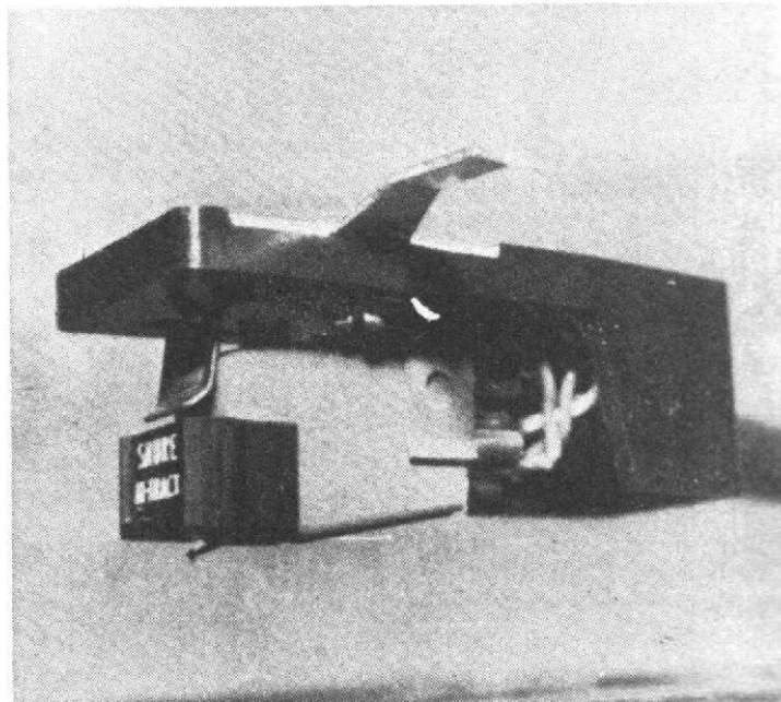
Fig. 19. — Porte-cellule Connoisseur permettant un réglage longitudinal de la position de la cellule.
