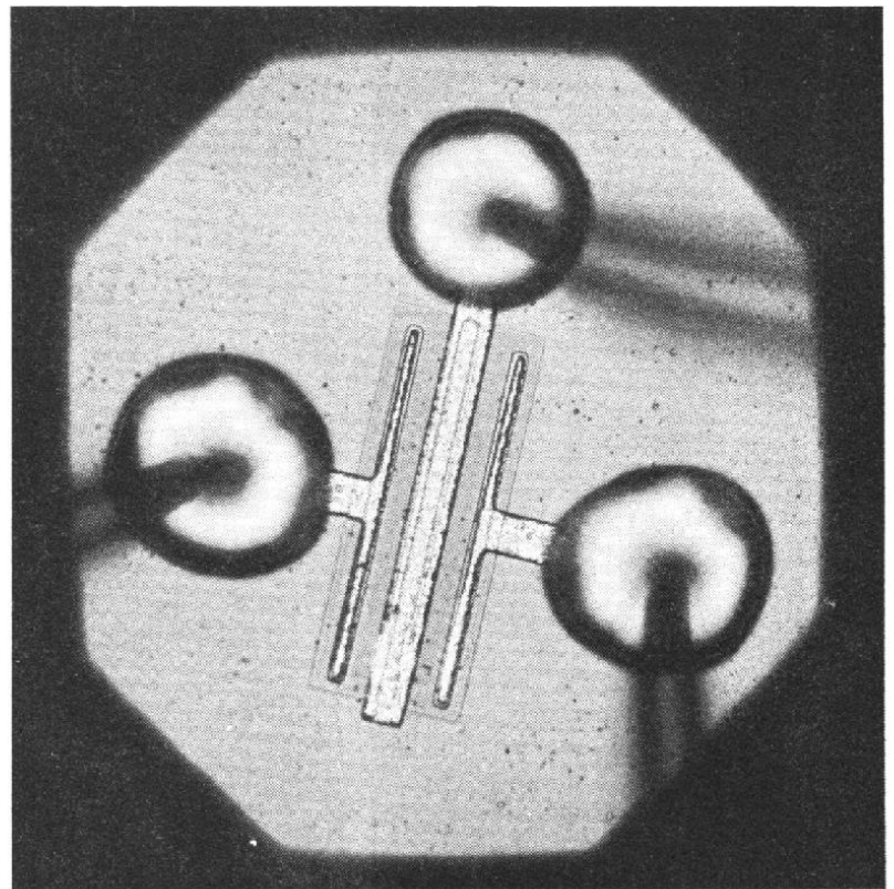
Fig. 3 Macrophotographie de la partie active d'un transistor MOS. Les masses sont les points de soudure des fils de sortie.
