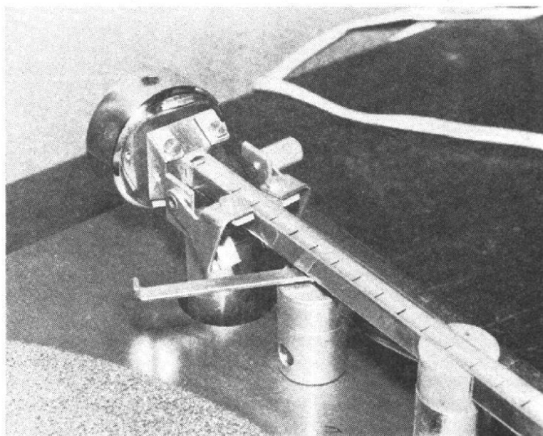
Fig. 13. — Vue du bras ERA à pivot fictif.
