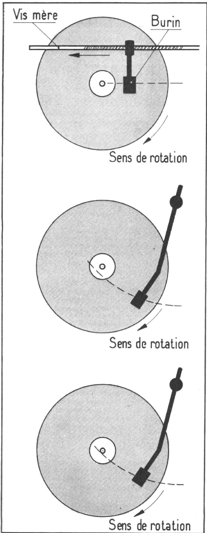
Fig. 1-2-3. — Rayon suivi par le burin et arcs de cercle décrits par les pointes de lecture.
