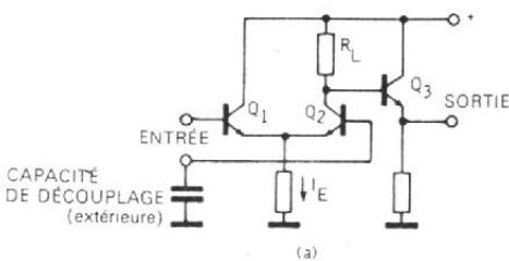
Fig. 2. - Schéma de l'un des trois étages de l'ampli-limiteur du TAA 661.
