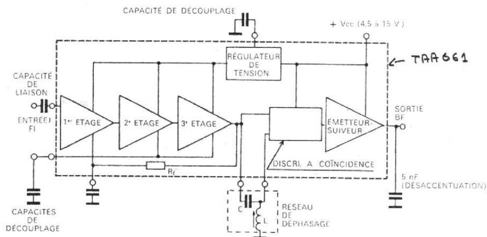
Fig. 1. - Bloc-diagramme du TAA 661.
