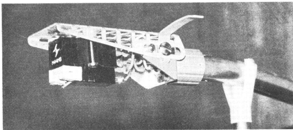
Fig. 18. — Porte-cellule Thorens avec dispositif de réglage longitudinal et vertical.
