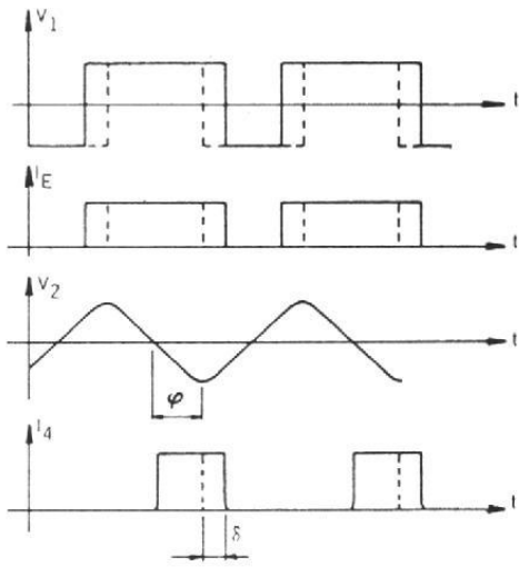
Fig. 6. - Le discriminateur demi-onde simple est sensible aux variations du rapport cyclique du signal ayant subi l'opération de limitation ( V_1 ).
