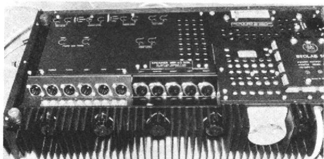
On notera l'importance des radiateurs des transistors de puissance et d'alimentation.
