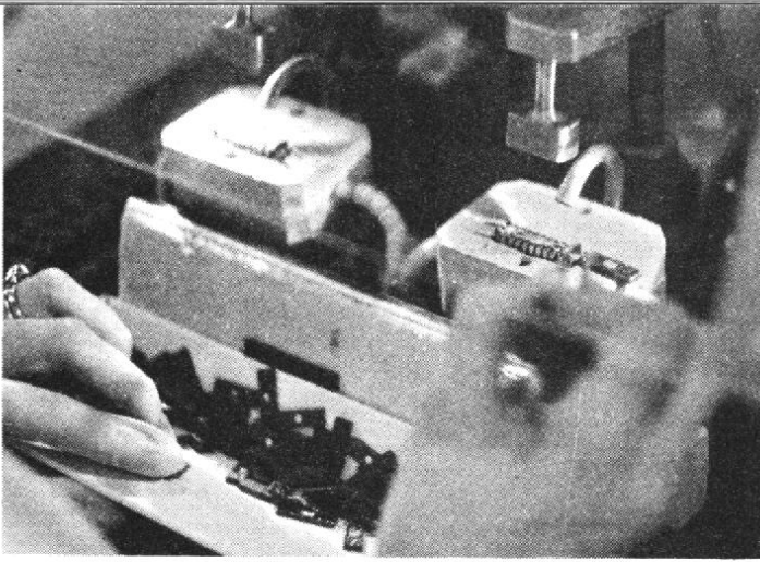
Cette machine permet l'encapsulation du circuit intégré. Les circuits Dual in line sont encapsulés par moulage.
