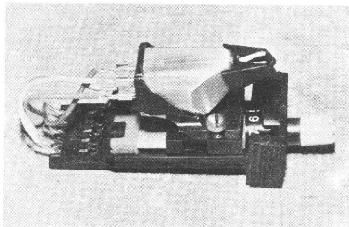
Fig. 22 a et b. — Porte-cellule P.E. avec dispositif de réglage d'angle d'attaque.
