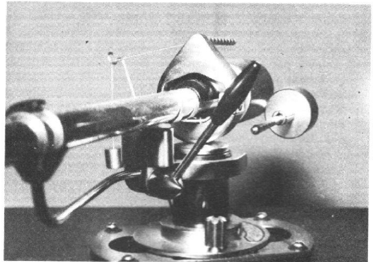
Fig. 16. — Pivot du bras S.M.E. (Cineco).
