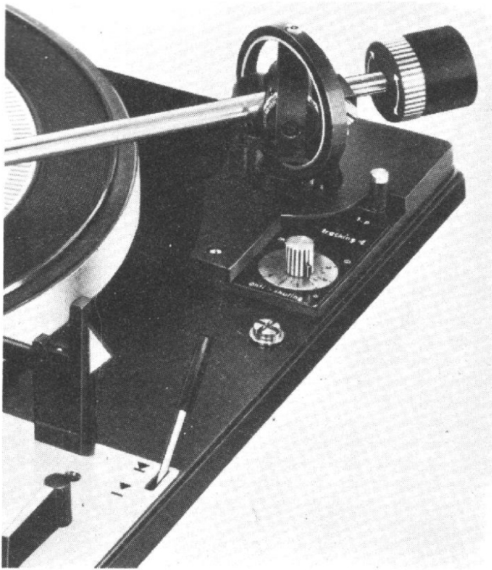
Fig. 14. — Pivot du bras Dual 1219.
