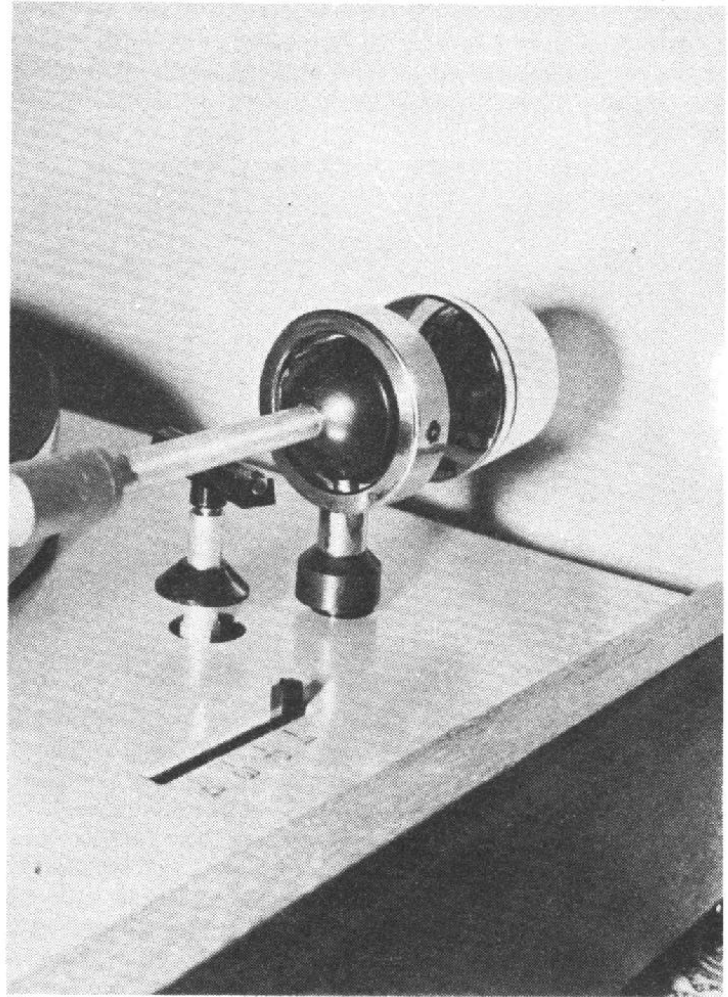
Fig. 15. — Pivot du bras Philips (202 et 208).
