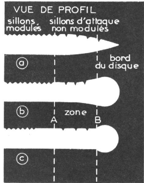
Fig. 11. — Coupe de bords des disques.
