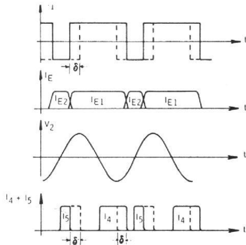
Fig. 8. - Le discriminateur demi-onde double est insensible aux variations du rapport cyclique de V_1 et aux perturbations, qu'en présence d'un signal V_1 dissymétrique (défaut dû au limiteur et causé essentiellement par les perturbations extérieures), le courant de sortie varie en plus ou en moins, ce qui modifie la valeur moyenne du courant. Cette sensibilité aux perturbations est éliminée par le
