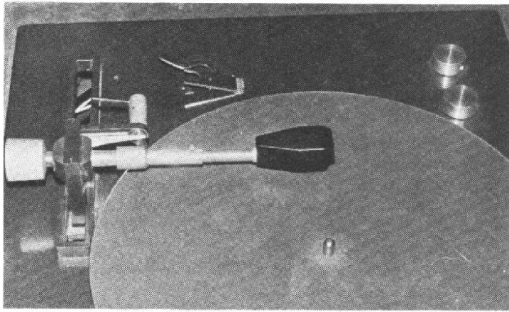
Fig. 6. — Bras Clément à déplacement radial asservi.
