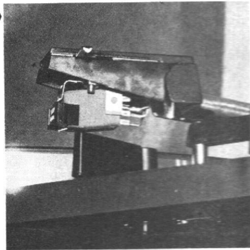
Fig. 20. — Dispositif à ressort pour la fixation des cellules Shure.
