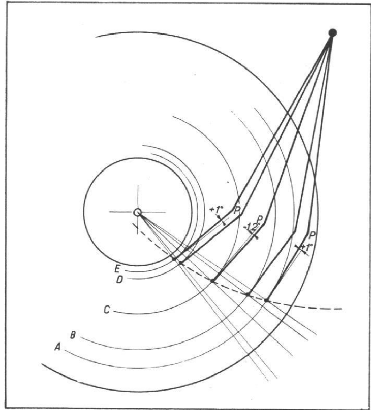
Fig. 7. — Méthode de détermination de l'angle d'erreur de piste.
