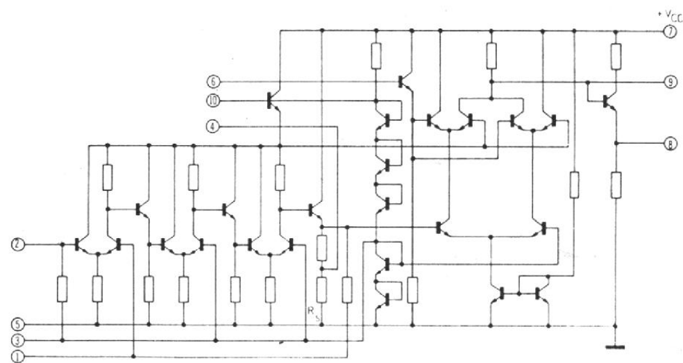
Fig. 4. - Schéma électrique du TAA 661.
