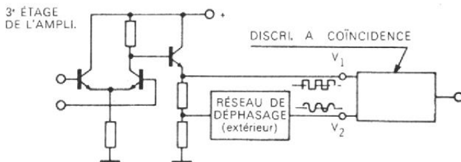
Fig. 3 - Principe de la liaison entre le 3 e étage de l'ampli et le discriminateur à coïncidence.
