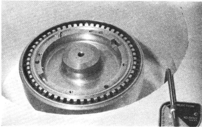
Etant donné les différentes formes sous lesquelles sont livrés les C.I., les essais de résistance mécanique ne sont pas faits dans un canon, mais avec un plateau tournant à très haute vitesse. Les C.I. sont placés dans les encoches. L'accélération atteint 20 000 G.
