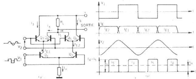
Fig. 7. - a) Discriminateur à coïncidence demi-onde double. b) Formes d'ondes sur ce type de discriminateur.
