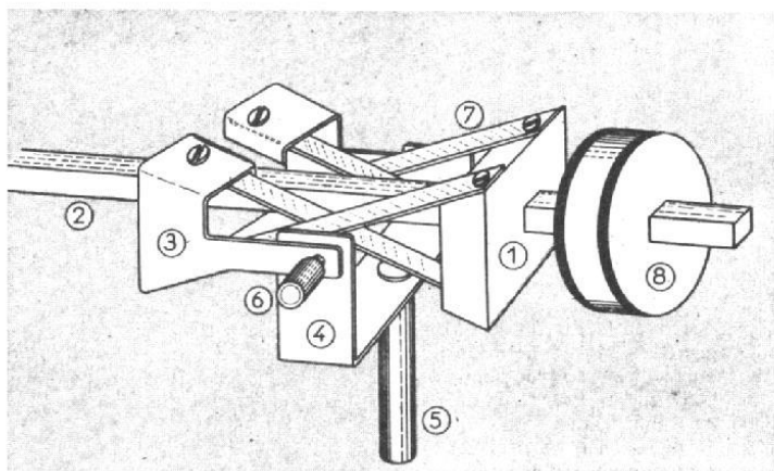
Fig. 12. — Schéma du bras ERA à pivot fictif.
