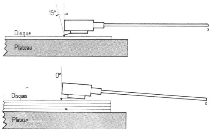
Fig. 21 a et b. — L'angle d'attaque de la pointe a été normalisé à 15°. Avec un changeur, cet angle est modifié par l'empilage des disques. Certains bras sont munis de dispositifs correcteurs (manuels).
