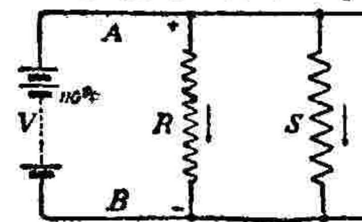
FIG. 34. — Représentation schématique du réseau d'éclairage électrique de la fig. 32. — V, tension électrique du réseau. A, B, fils positif et négatif du réseau ; R, S, résistances électriques des lampes. La résistance R, plus élevée que la résistance S, est représentée par un zig-zag plus rapproché qui la caractérise.
