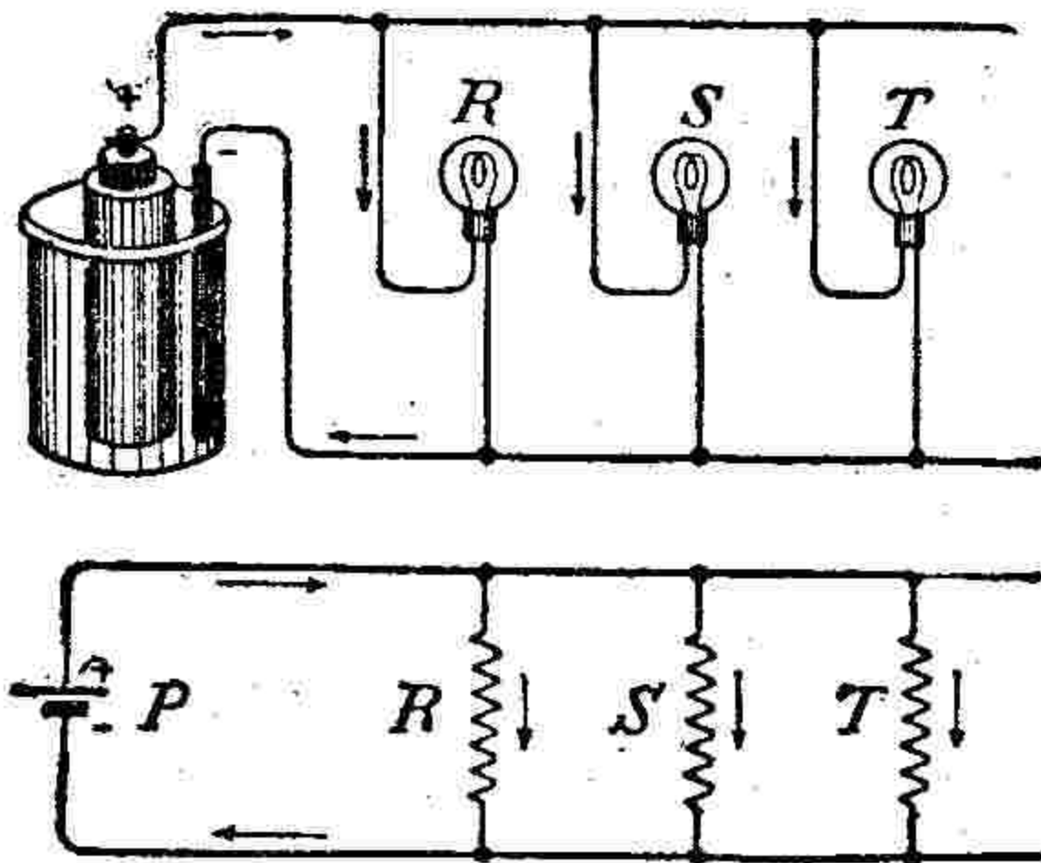
FIG. 35. — Comment l'on dispose des lampes en parallèle. — P, pile, source de courant ; R, S, T, lampes disposées chacune directement en dérivation ou en « parallèle » aux bornes du réseau. Les courants traversant les 3 lampes s'ajoutent dans les conducteurs généraux du réseau. L'inverse des résistances de chacune des lampes s'ajoute ainsi pour donner la valeur de l'inverse de la résistance de l'ensemble.
