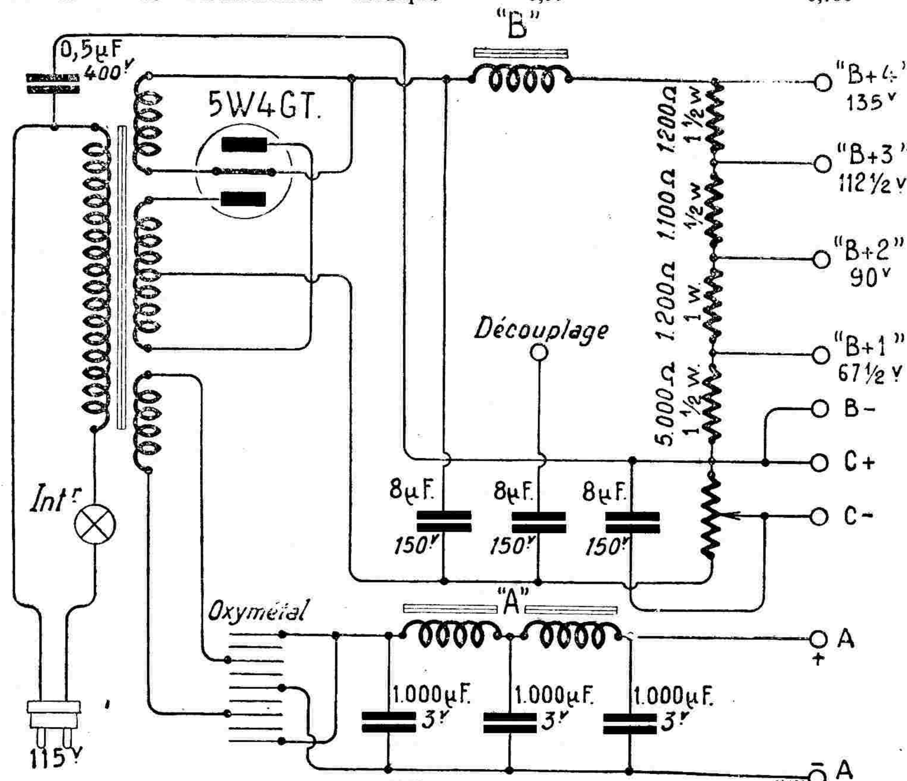
Schéma de principe de la boîte d'alimentation pour poste à batteries transformé
