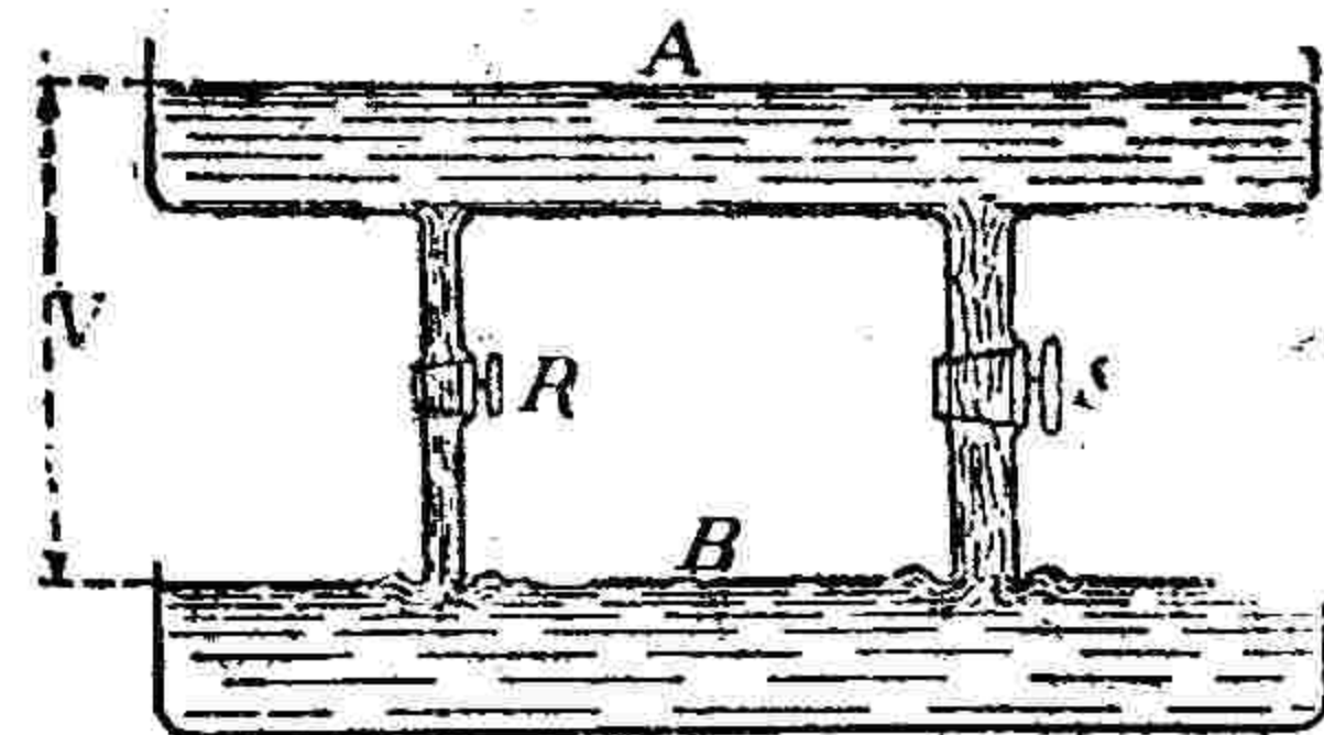
FIG. 33. — Analogie hydraulique du réseau électrique d'éclairage de la fig. 32. — A, B, réservoirs d'eau supérieur et inférieur, analogues aux fils positif et négatif du réseau. R, S, canalisations, l'une étroite, l'autre large, analogues aux résistances électriques, l'une élevée, l'autre moindre des lampes R et S. V, différence de niveau d'eau analogue à la différence de niveau ou tension électrique entre les deux fils positif et négatif du réseau.
