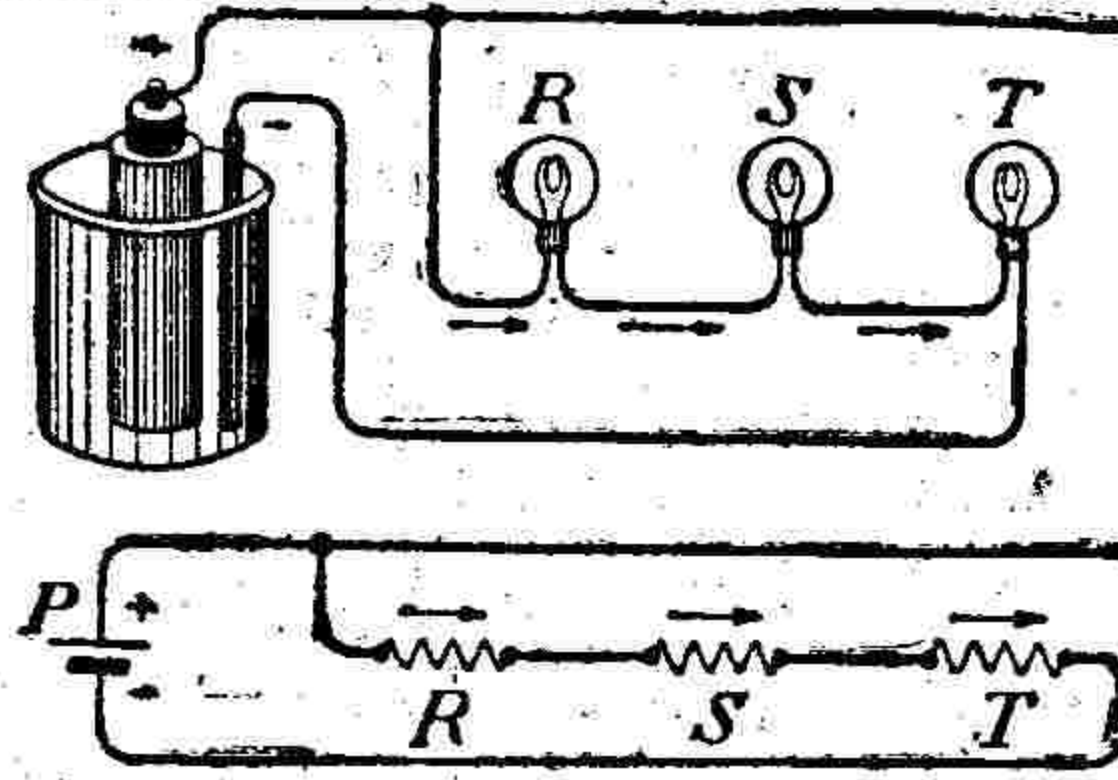
FIG. 36. — Comment l'on dispose des lampes en série. — P, pile alimentant le réseau; R, S, T, lampes associées en série, c'est-à-dire connectées à la suite les unes des autres. Les résistances s'ajoutent en série et la résistance totale est égale à la somme des résistances élémentaires de chacune des lampes.
