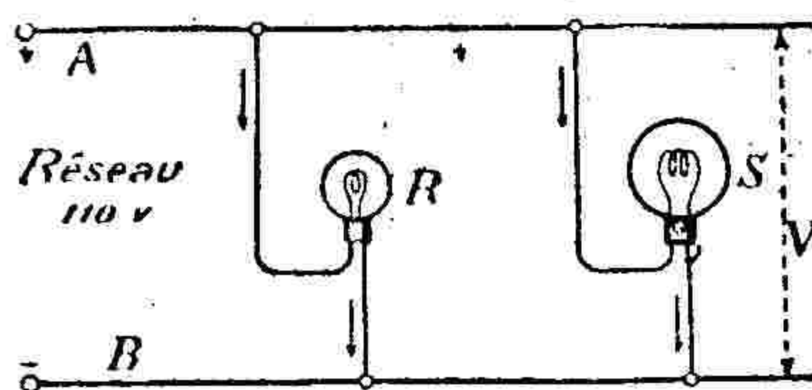
FIG. 32. — Représentation d'un réseau d'éclairage électrique. — Entre les deux fils A (positif, et B (négatif) du réseau, on place des dérivation composées de 2 fils de connexion aboutissant aux lampes R et S de résistances différentes.
