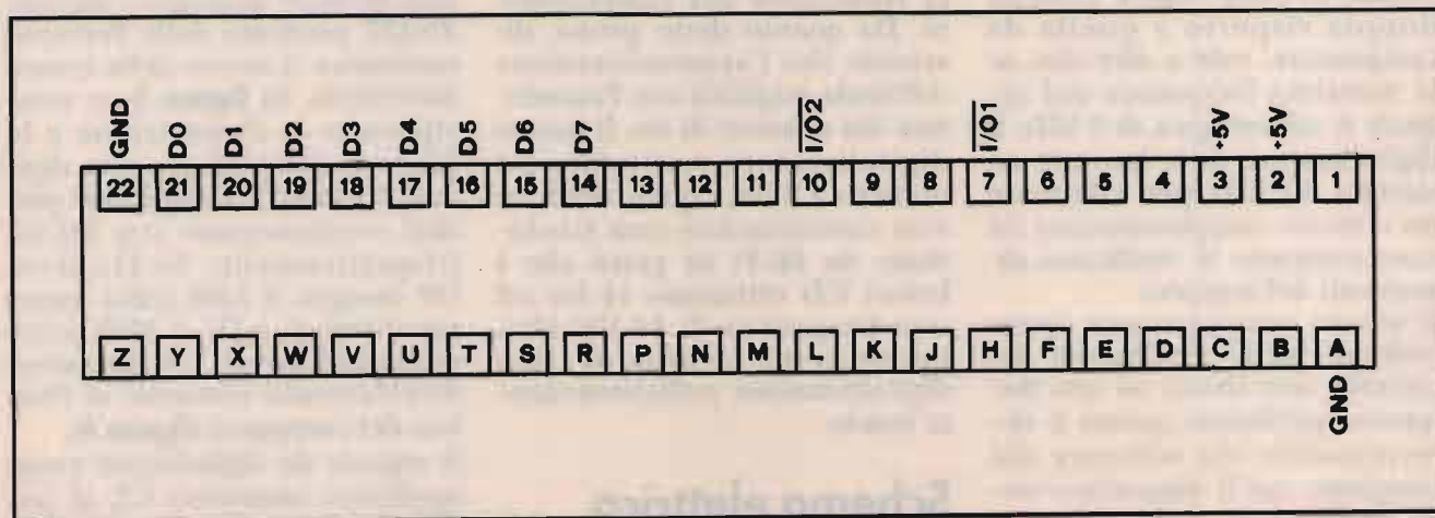
⑥ Connessioni e relative funzioni della EXPANSION PORT del C64 (vista frontale).
