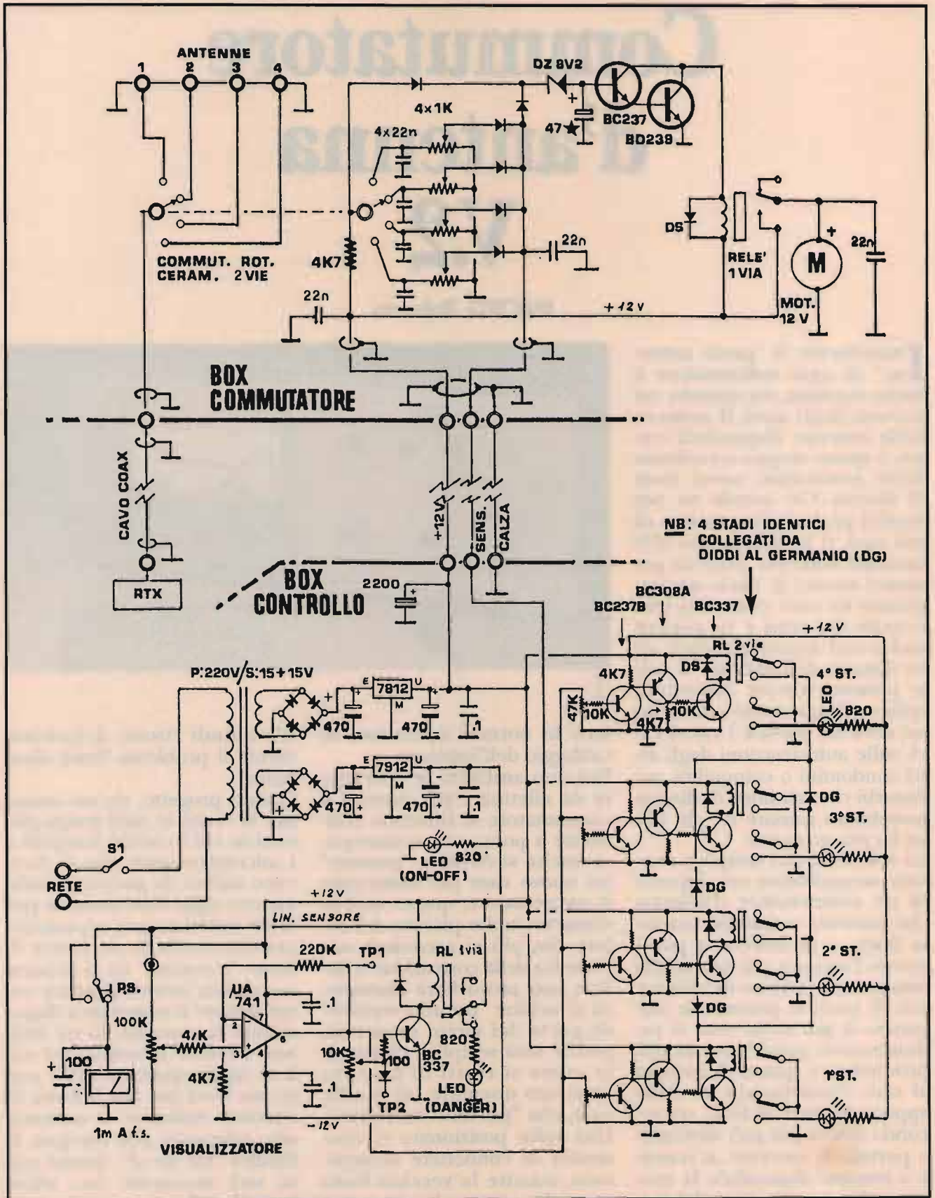
② Schema elettrico generale.
