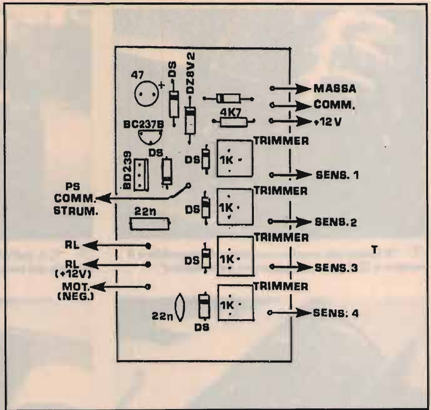
8 Posizionamento componenti sul C.S. del sensore di posizione.
