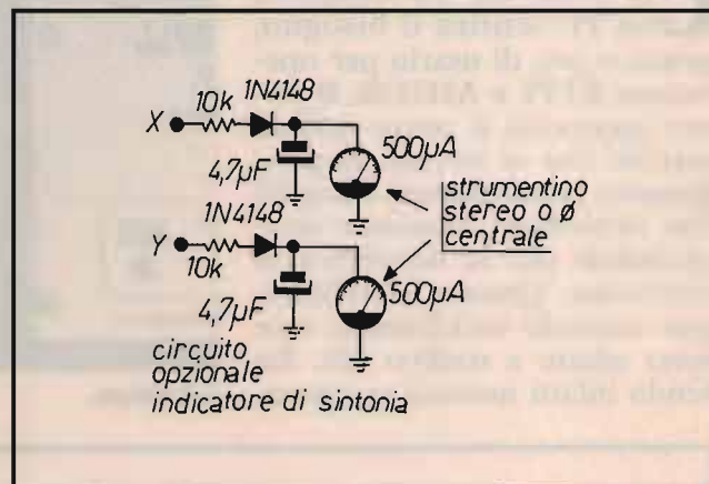
⑤ Circuito opzionale indicatore di sintonia.
