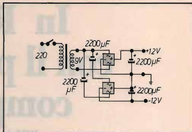
③ Alimentatore duale.
