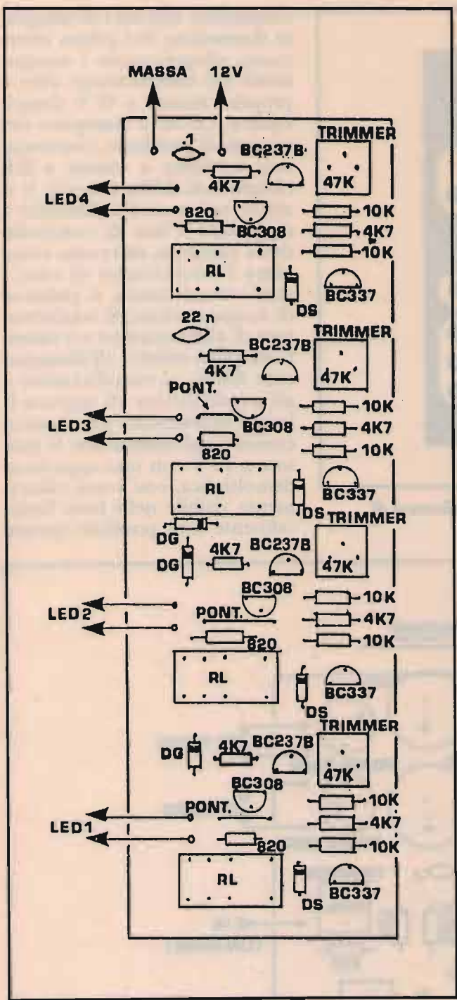
③ Posizionamento componenti sul c.s. del visualizzatore.
