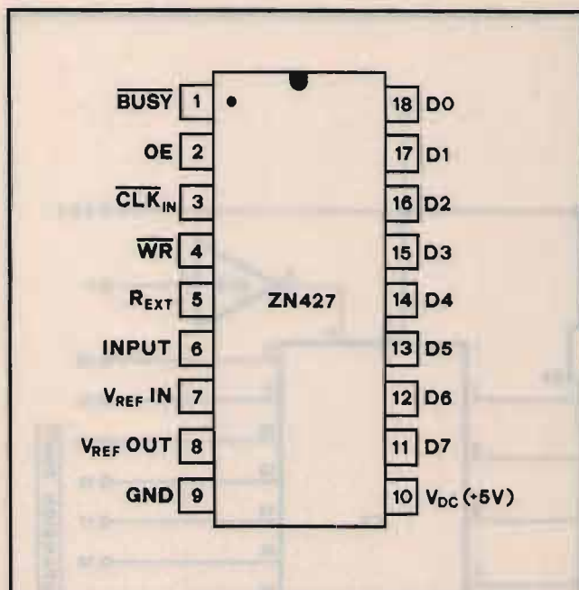
⑤ Connessioni dei circuiti integrati utilizzati e relative funzioni.
