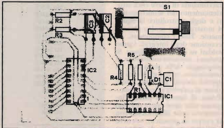
4 Disposizione dei componenti sul circuito stampato.
