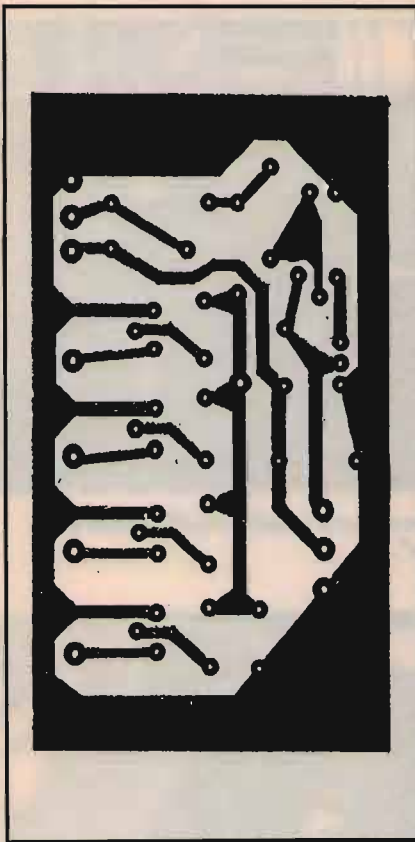
7 C.S. del sensore di posizione.
