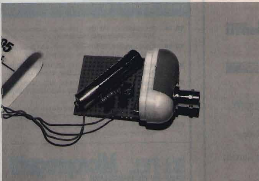
Circuito interno.
