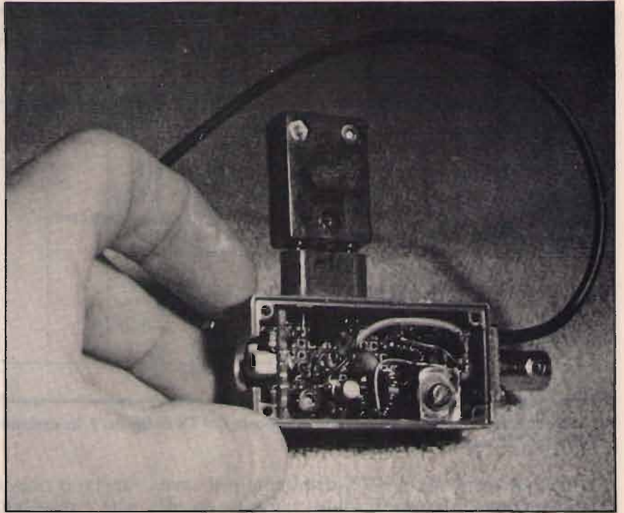
③ Il montaggio del TX, date il minimo spazio disponibile, è del tipo punto-a-punto; un ritaglio di millefori rappresenta il supporto generale del tutto.
