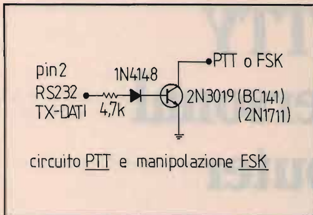
② Circuito PTT e manipolazione FSK.
