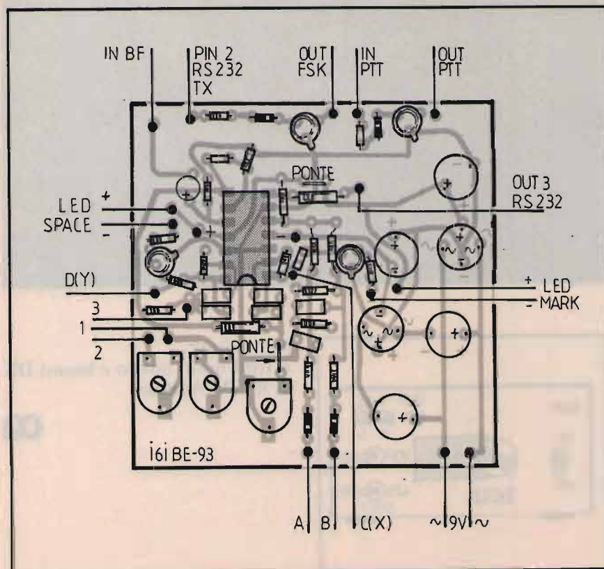
⑦ Disposizione componenti.
