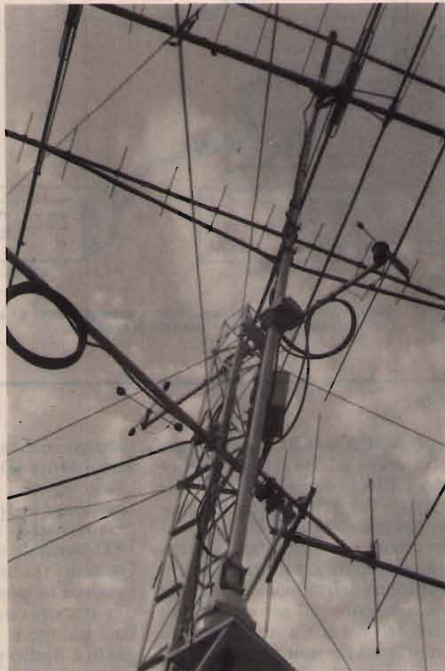
⑯ Posizionamento del Box-commutatore alla sommità del traliccio".
