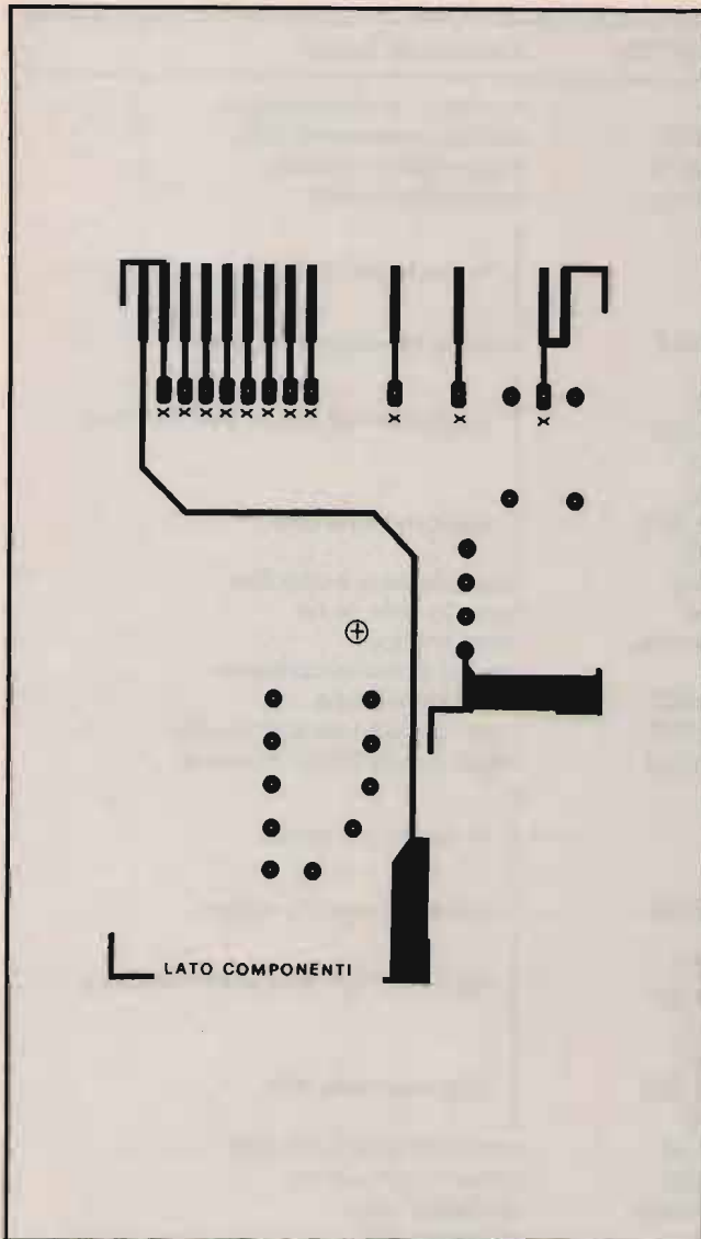
3a Circuito stampato scala 1:1 (lato componenti).
