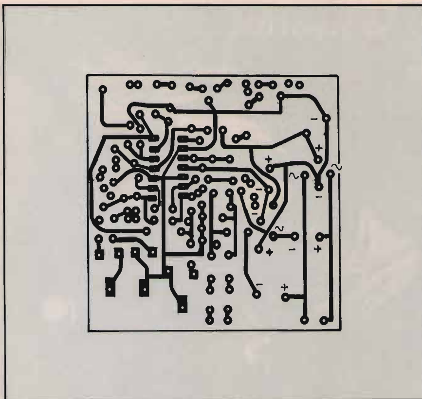
⑥ Lato rame RS232 scala 1:1.
