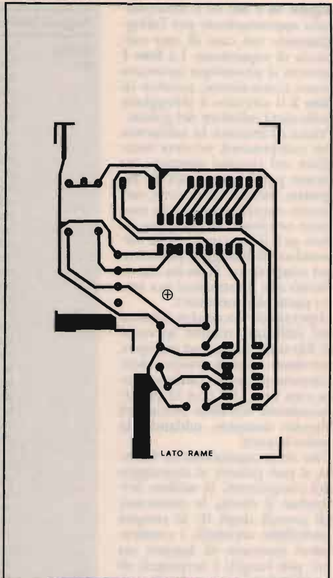
3b Circuito stampato scala 1:1 (lato saldature).
