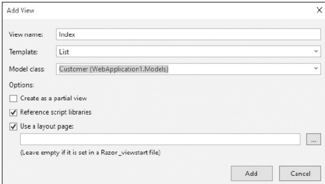
Figura 16.8 – Creare una view tipizzata con ASP.NET MVC.
