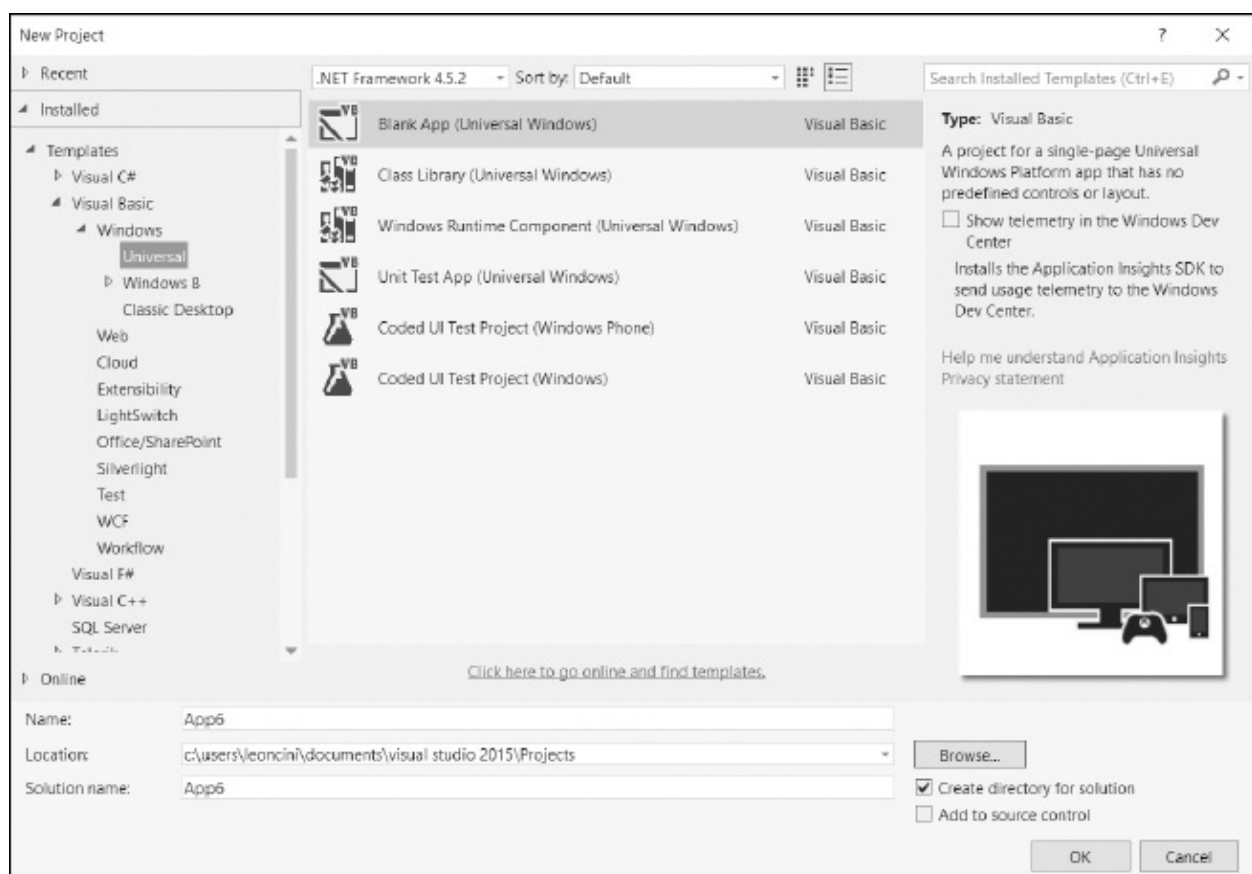
Figura 15.1 – I progetti aggiuntivi per creare applicazioni Universal Windows Platform offerti in Visual Studio 2015.
