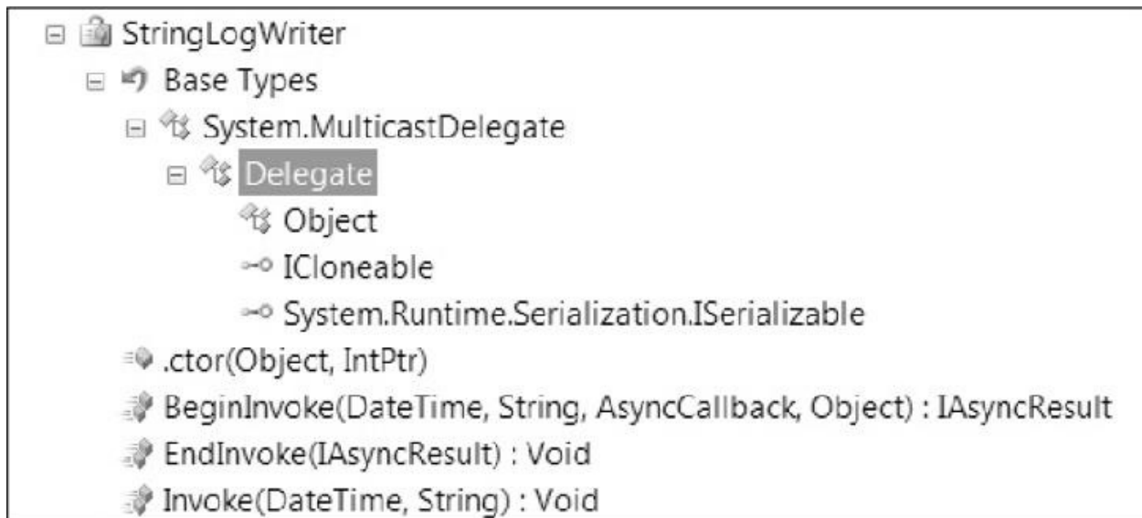
Figura 6.2 – Gerarchia di StringLogWriter.
