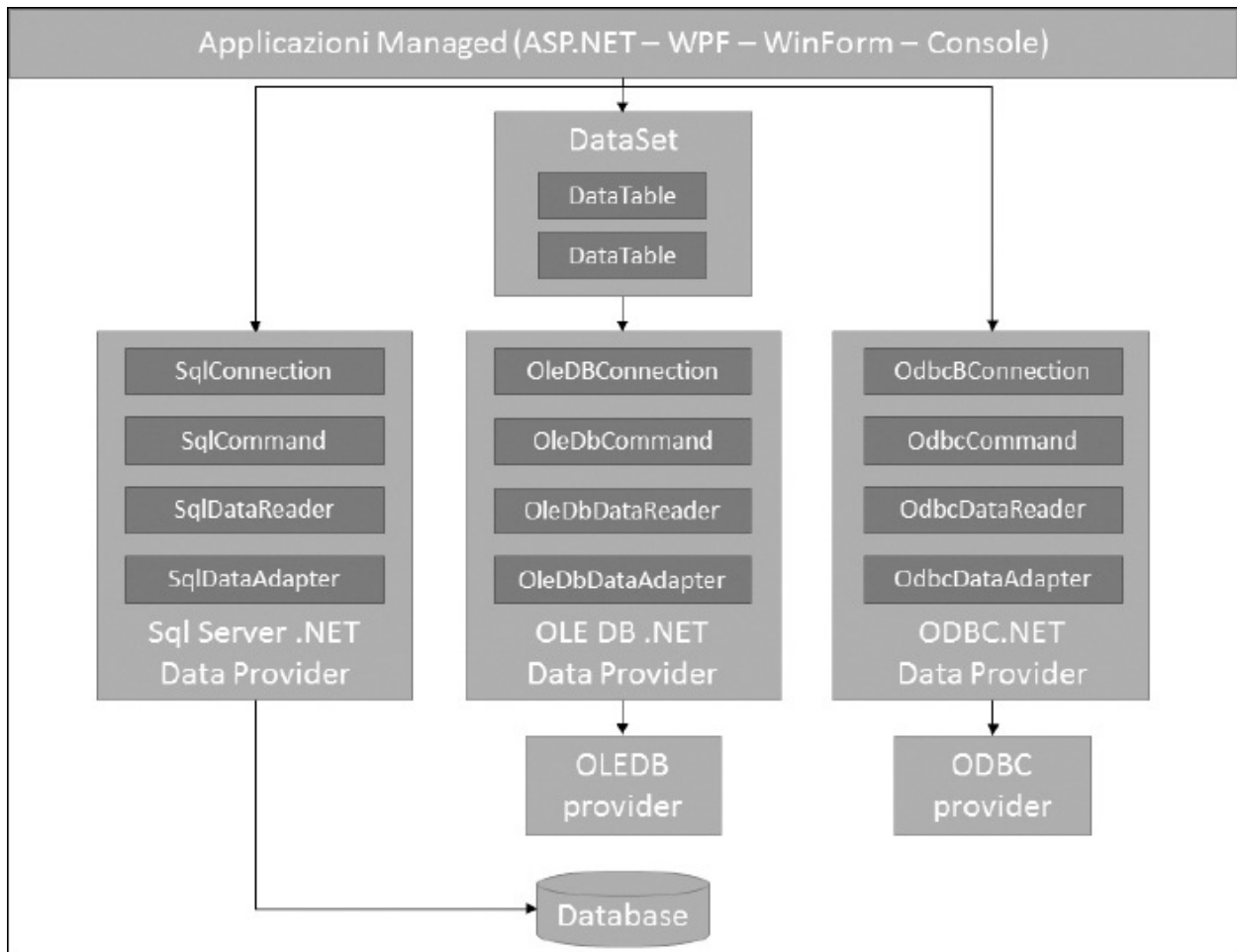
Figura 10.1 – Architettura di ADO.NET.
