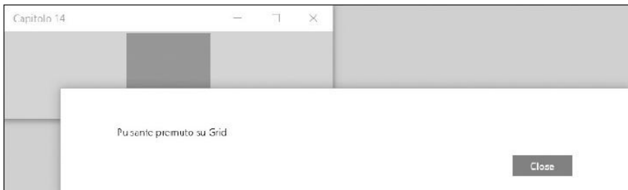
Figura 14.8 – La propagazione degli eventi intercettata e mostrata attraverso una MessageBox.
