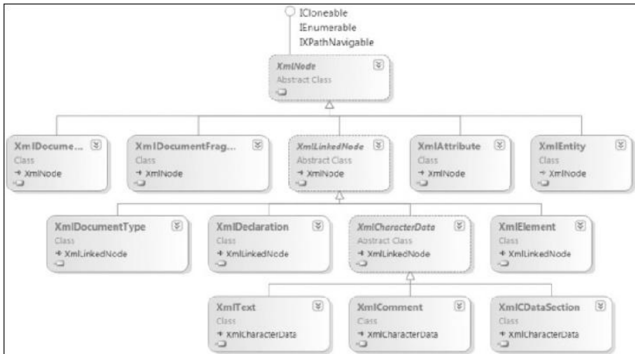
Figura 12.2 – Struttura gerarchica delle classi System.Xml.
