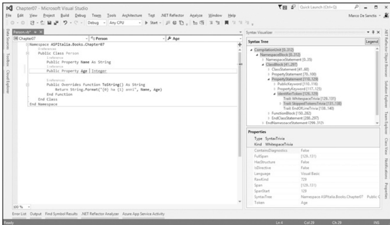
Figura 7.7 – Errore di sintassi nel Syntax Visualizer.
