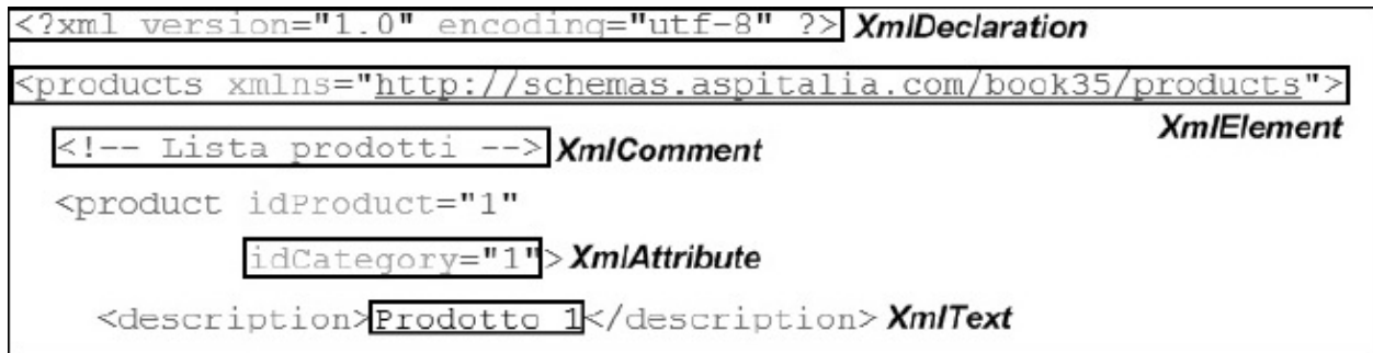
Figura 12.1 – Frazionamento di un documento XML secondo DOM.
