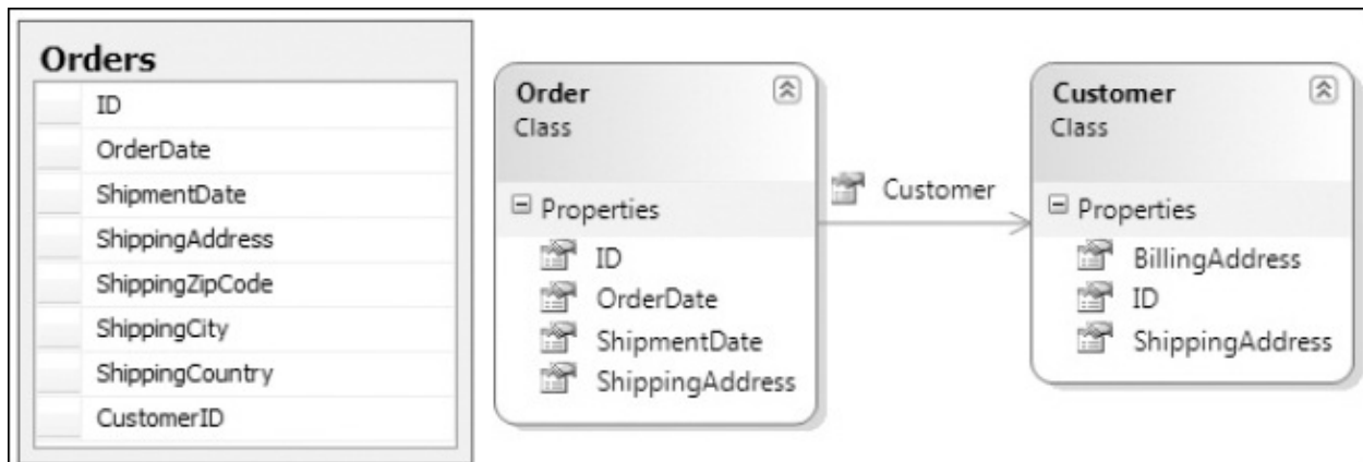
Figura 11.2 – La relazione tra ordini e clienti è mantenuta con una foreign key sul database e con una proprietà sul modello.
