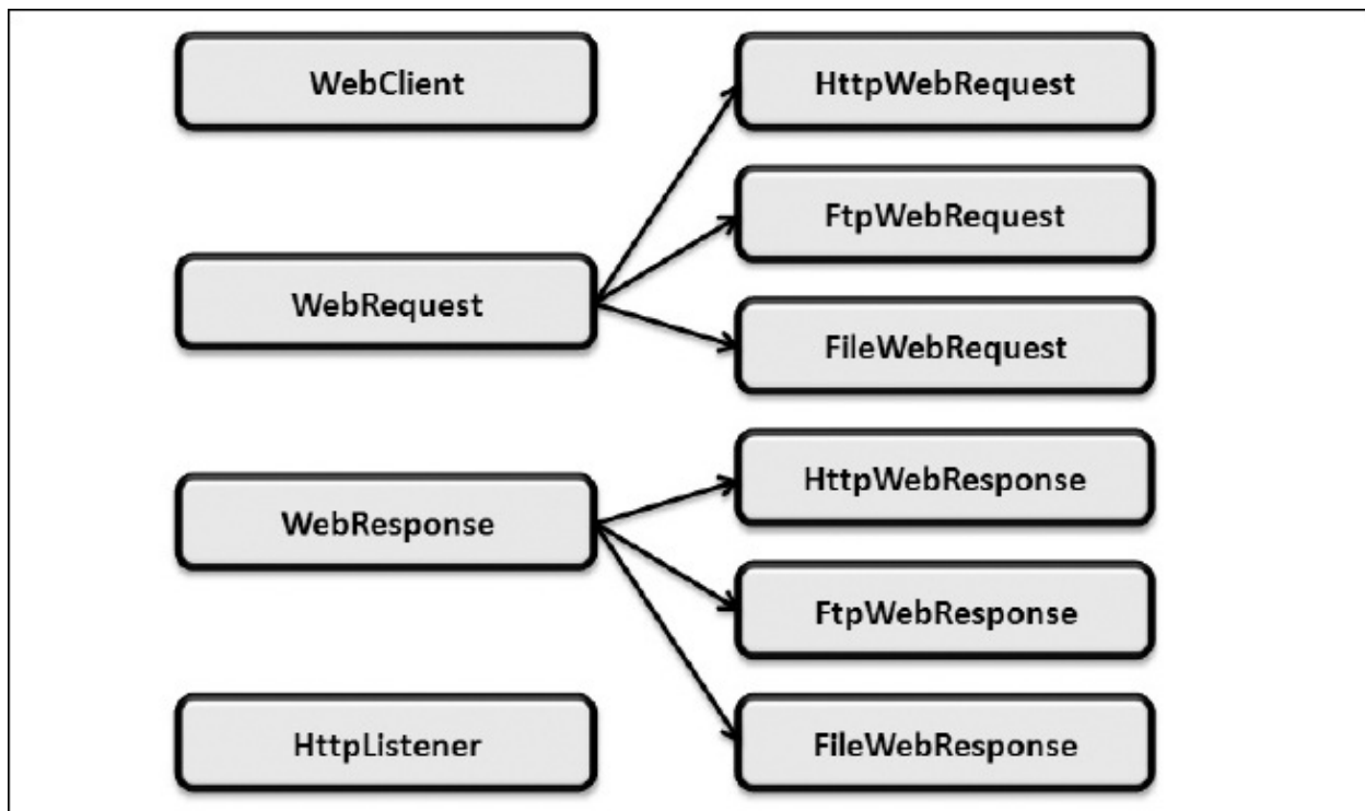
Figura 19.12 – Gerarchia degli oggetti namespace System.Net.
