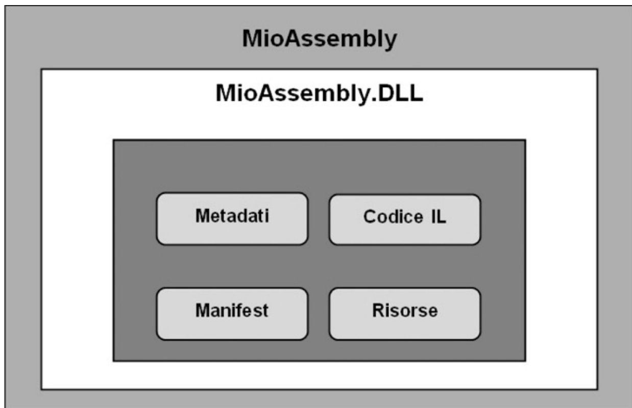
Figura 1.4 – Lo schema semplificato di un assembly.
