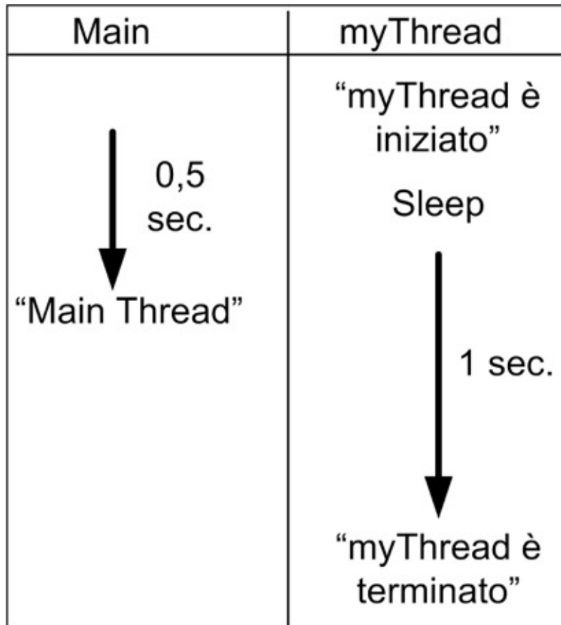
Figura 9.2 – Parallelismo dei thread dell'esempio 9.1.
