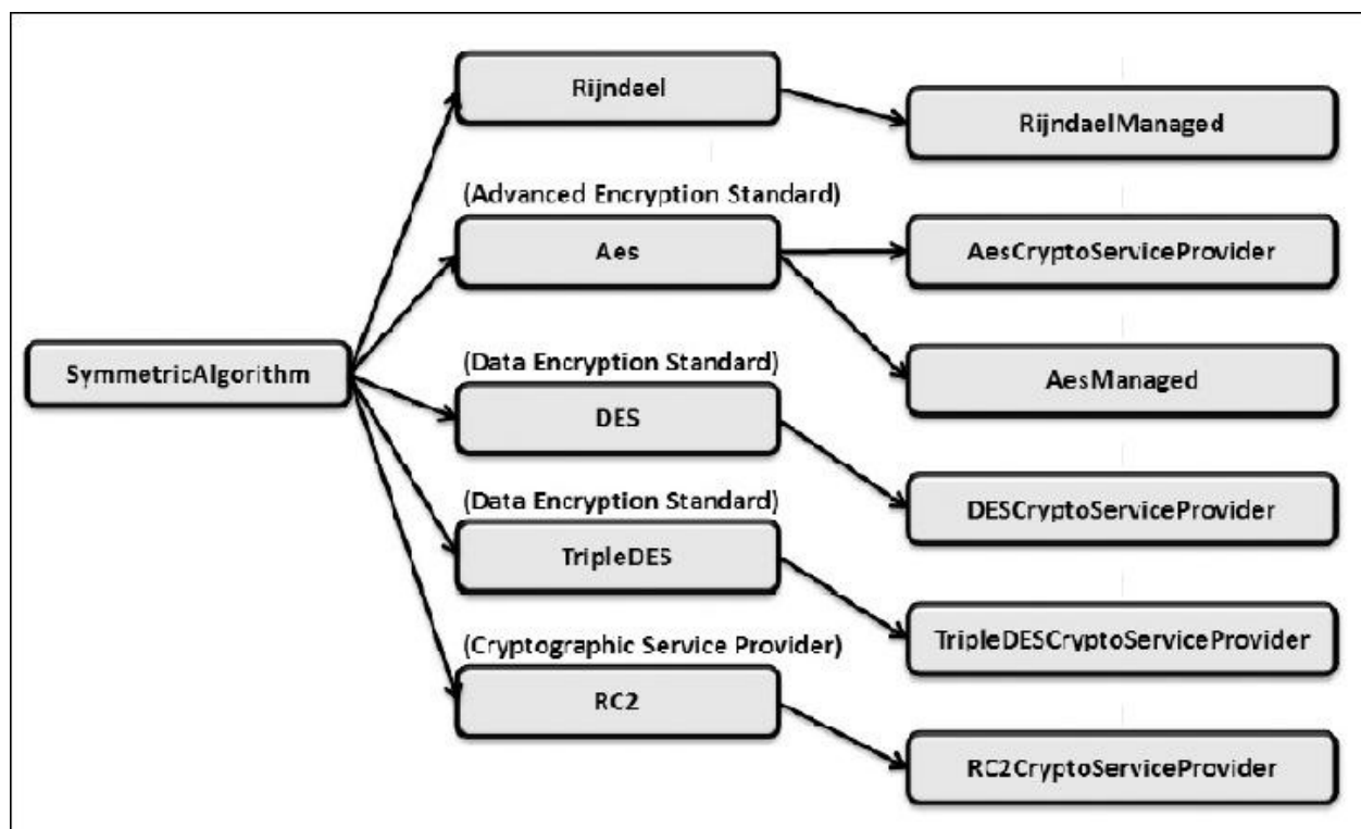
Figura 18.2 – Gerarchia delle classi SymmetricAlgorithm.
