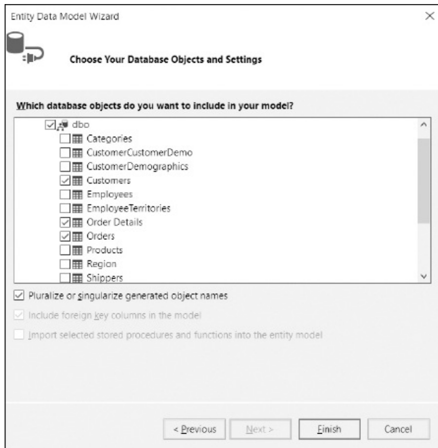
Figura 11.5 – La maschera per selezionare gli elementi del database da mappare.
