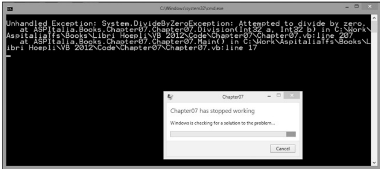
Figura 7.1 – Applicazione terminata per eccezione non gestita.
