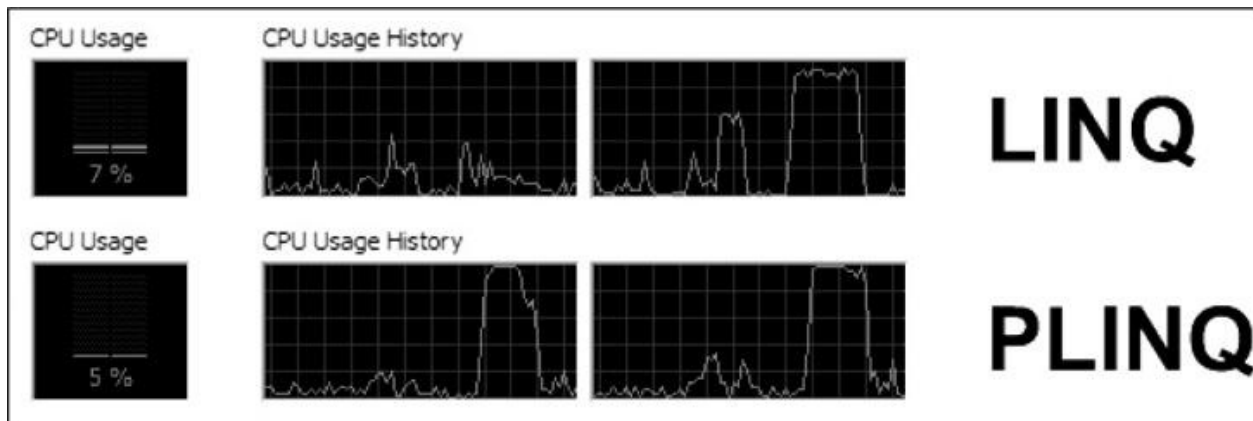
Figura 9.4 – Utilizzo delle CPU senza e con PLINQ.
