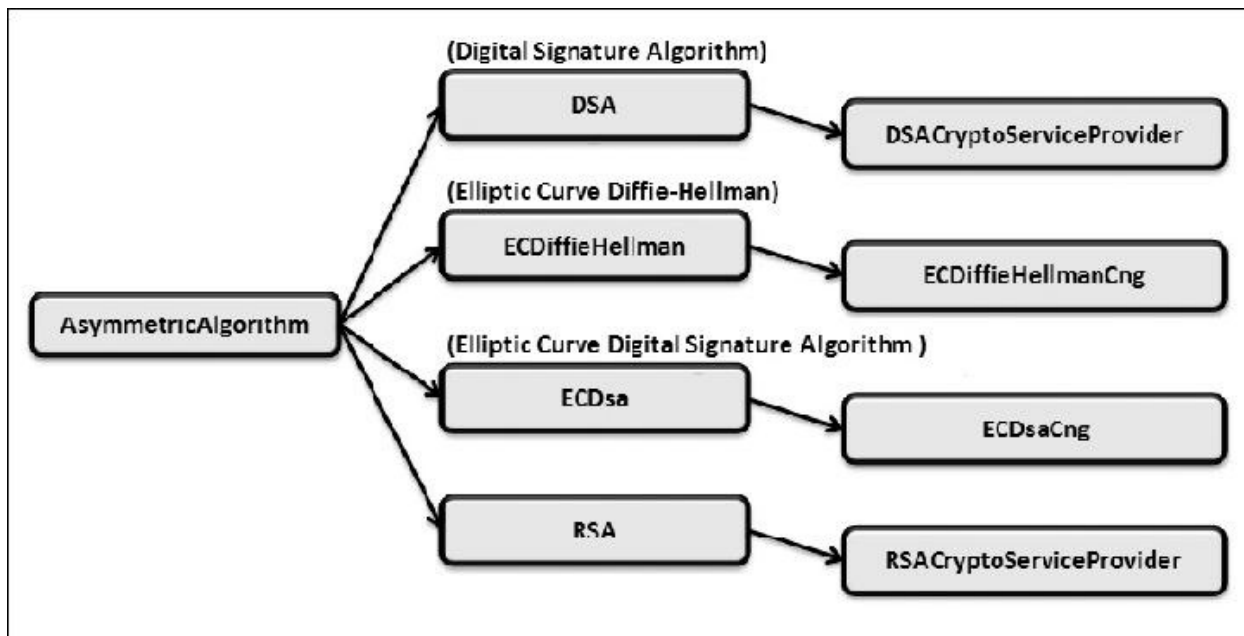
Figura 18.3 – Gerarchia delle classi AsymmetricAlgorithm.
