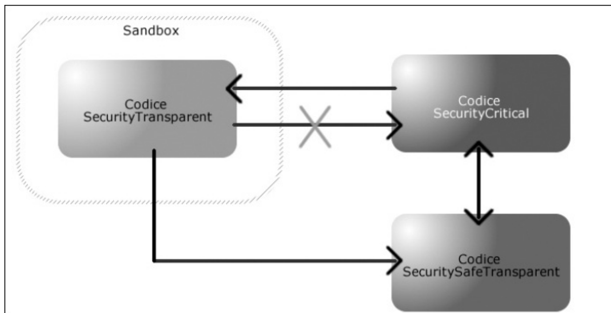
Figura 18.1 – Accesso al codice nel Level 2 Security Transparency model.
