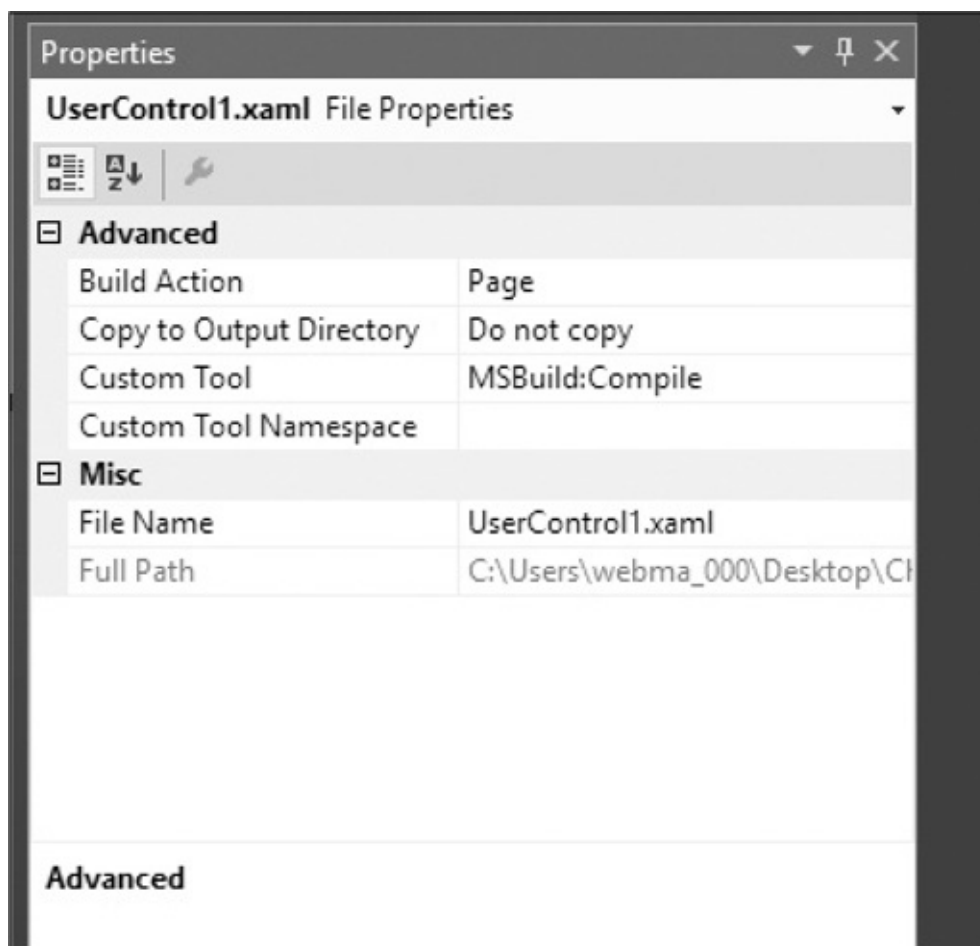
Figura 2.5 – Il Property Editor di Visual Studio.
