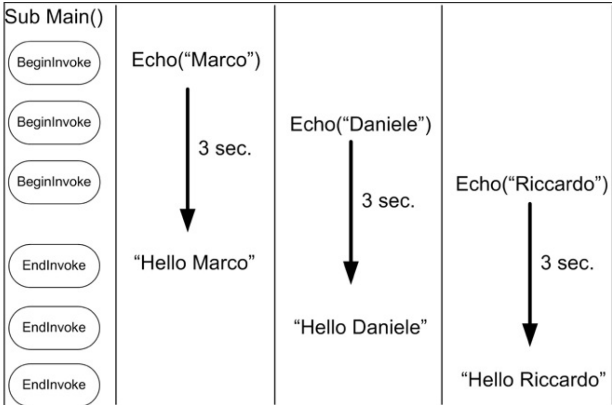
Figura 6.5 – Schema di esecuzione multithreaded.
