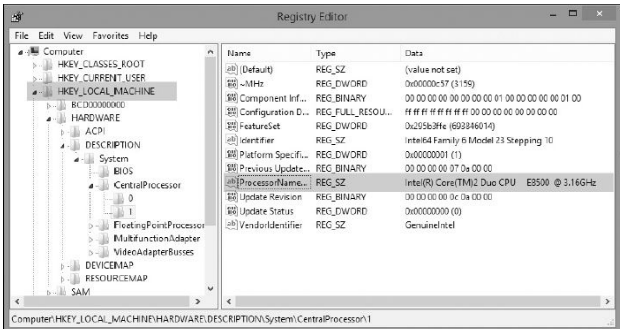
Figura 19.7 – L'applicazione RegEditor.
