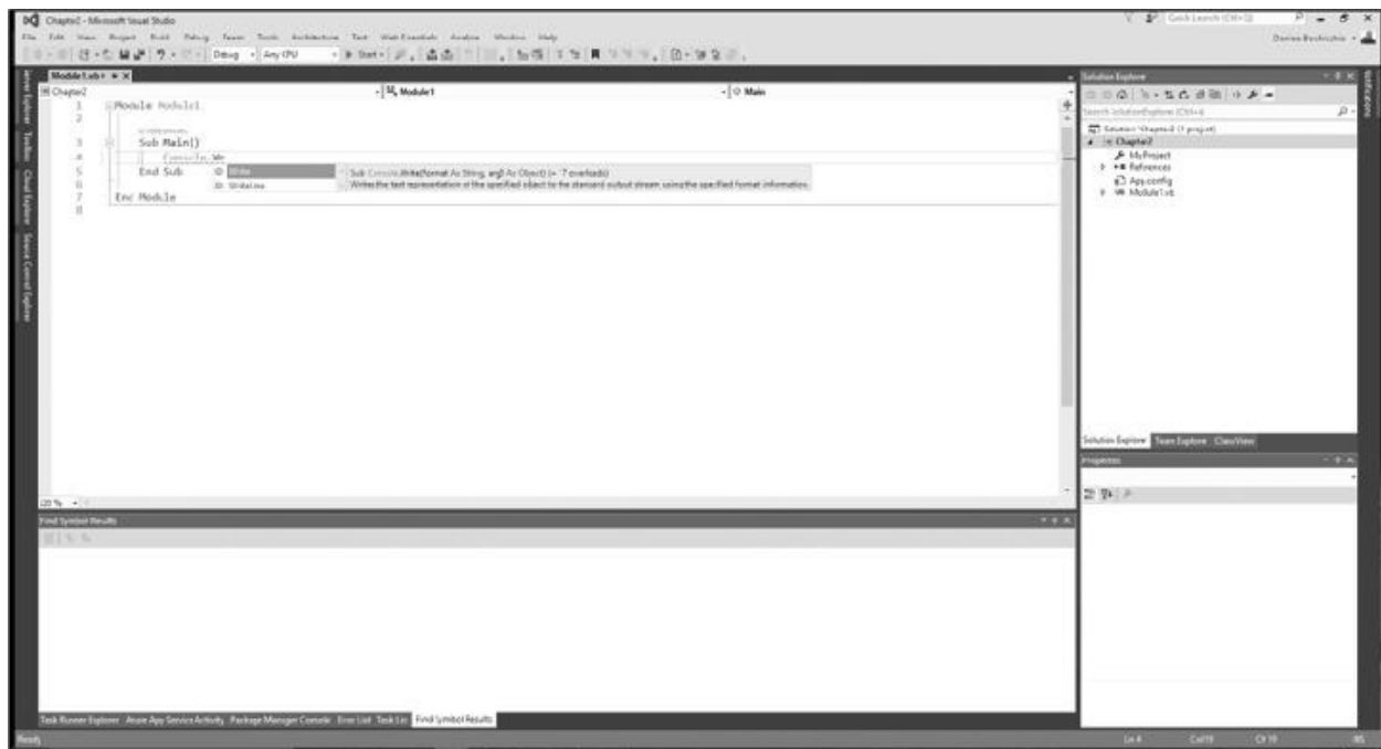
Figura 2.2 – L’Intellisense all’opera.
