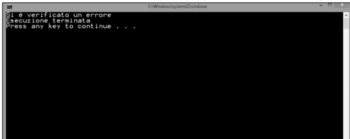
Figura 7.3 – Eccezione gestita.
