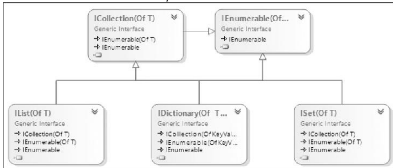
Figura 5.4 – Interfacce delle collection generiche.
