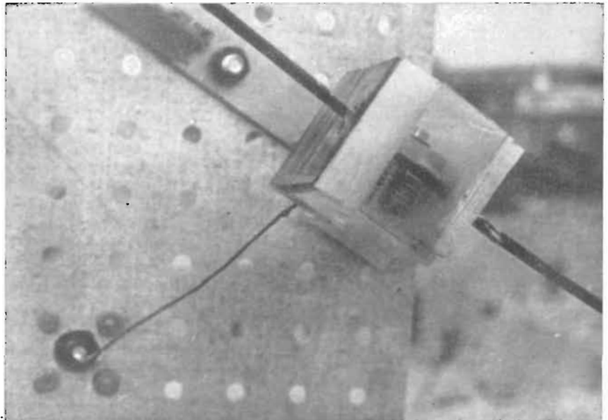
Figura 115 Particolare del « Gamma match ».
