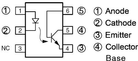
4N35 U17
