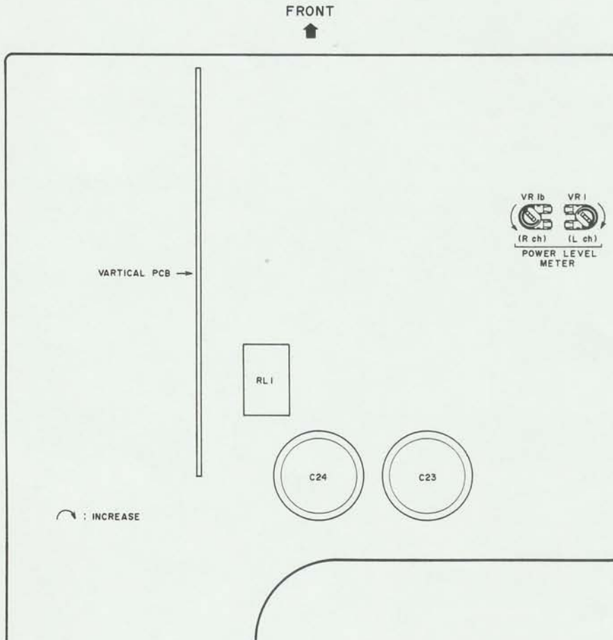
Fig. 6-2 Main-Amp PCB
