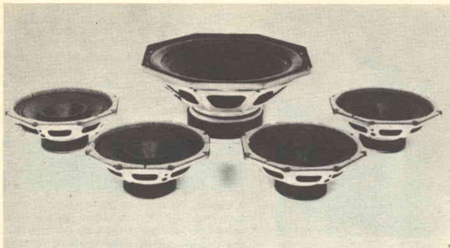
Presentazione degli altoparlanti usati nel "Più 4": un woofer a sospensione di butile e quattro tweeter biconici.
