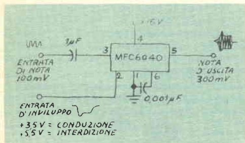
Fig. 5 - Sagomatore di involuppo a blocco di guadagno.
