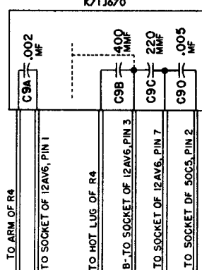
Bulbplate Connectors
