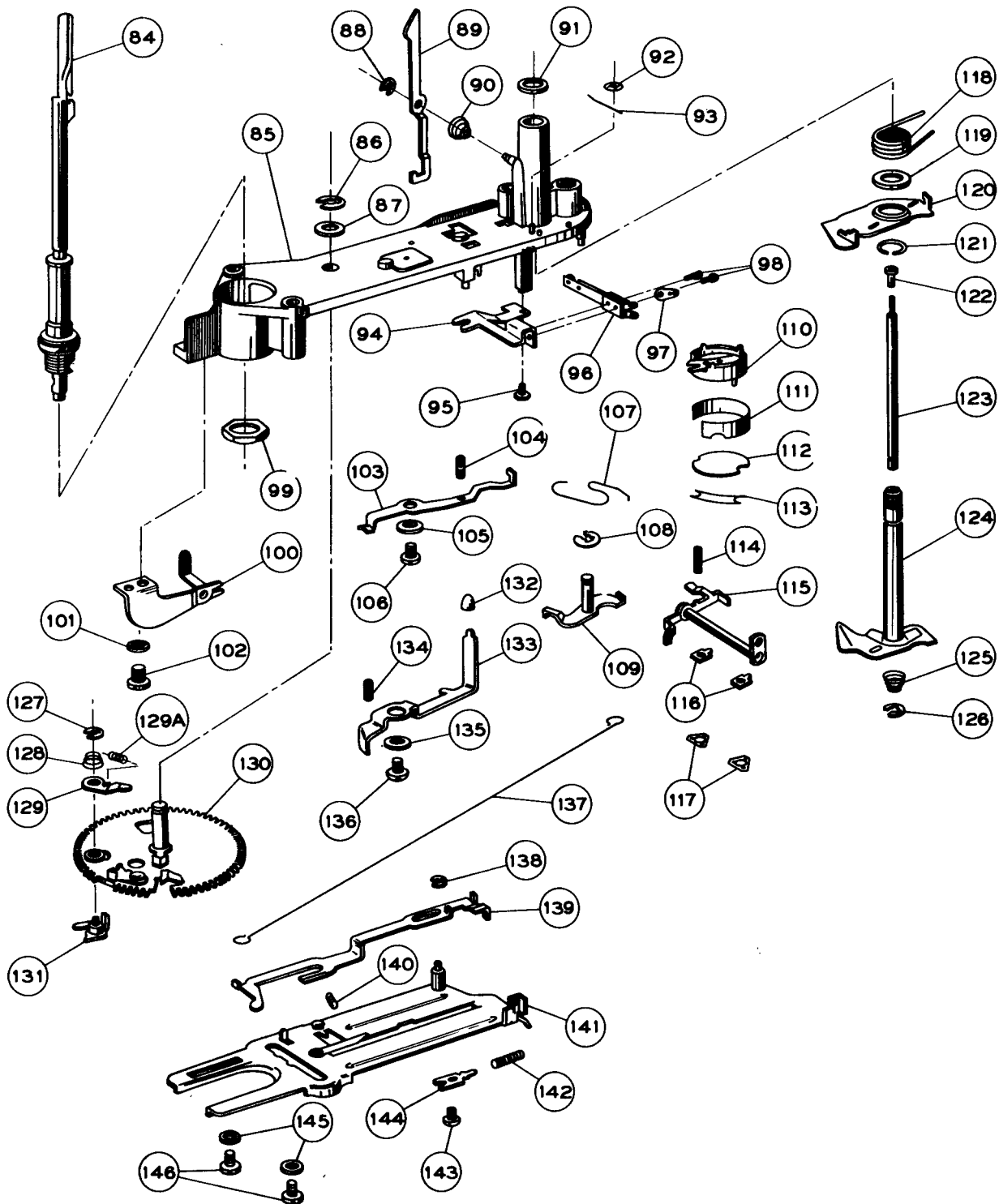
Fig. 27—Slide Assembly
