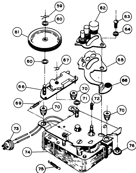
Fig. 28—Motor Assembly
