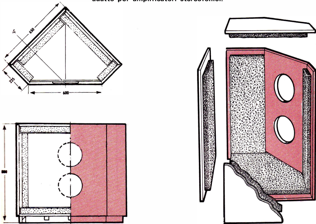
Fig. 9 MOBILE «PENTAGONALE». adatto per amplificatori stereofonici.
