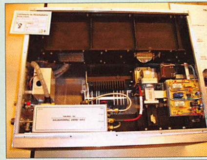
5 - Transverter 70/3 cm, 50 W HF, par F5BUU.
