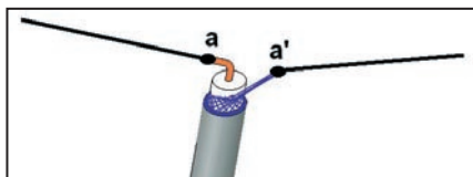
Figure 5: Raccordement d'un câble coaxial à un dipôle.
