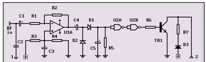
Figure 1 - Commutation par un signal BF.
