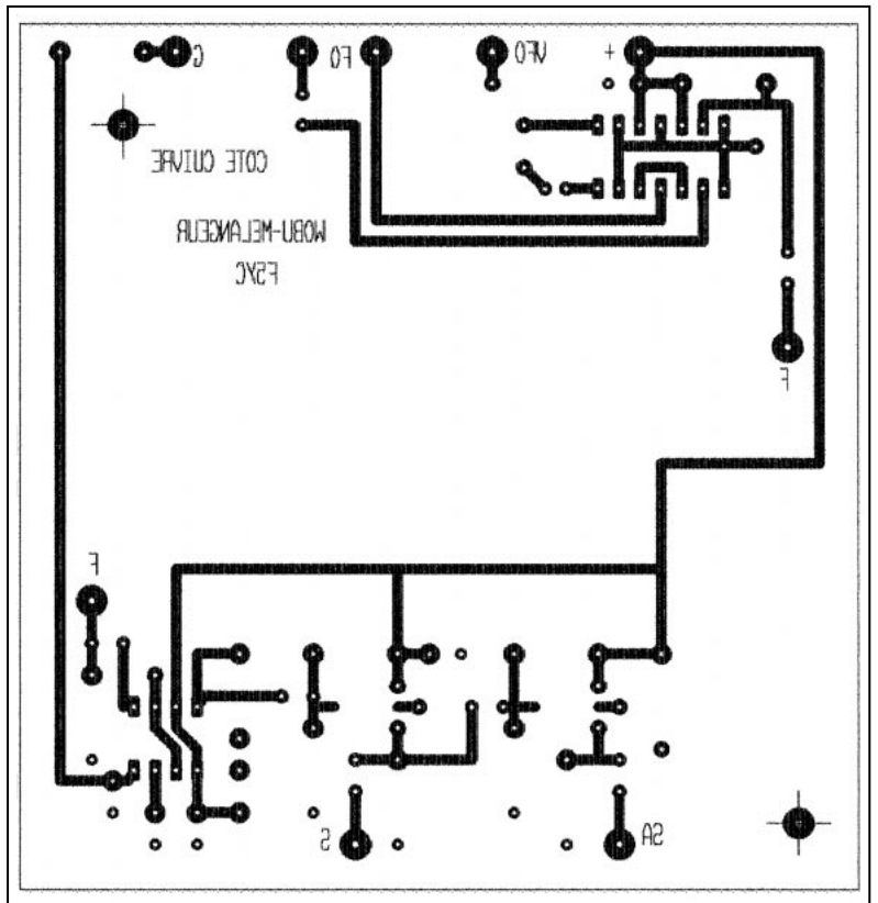
CI.4 Wobulateur 0,5-45 MHz.
