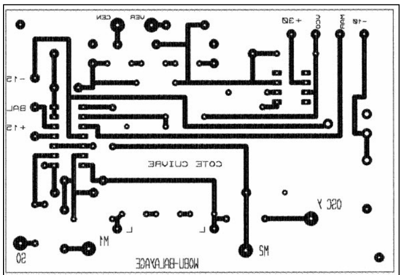
CI.5 Wobulateur 0,5-45 MHz.
