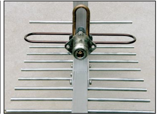
Antenne WiMo.
