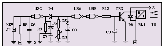
Figure 2 - Manipulation temporisée.
