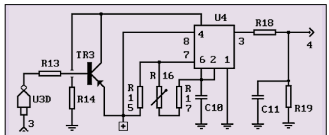
Figure 3 - Oscillateur.
