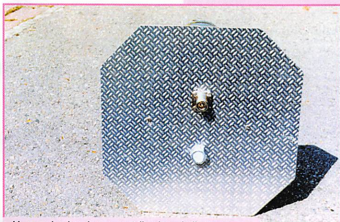
Vue sur le plan de masse à l'arrière de l'antenne. Diamétralement opposés, la fiche N et la vis Nylon.
