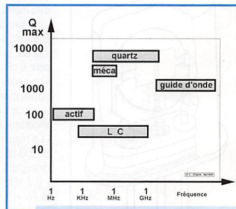
Schéma 3 : Fréquence d'utilisation et Q maximum de filtres passe-bande selon la technique employée.
