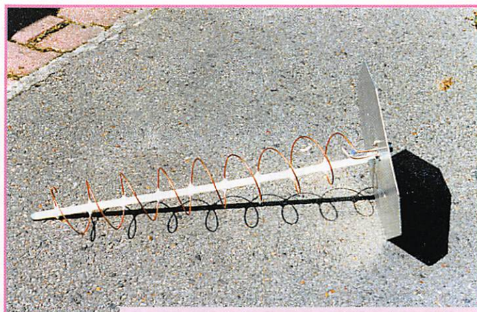
Vue générale de l'antenne sans son capot.
