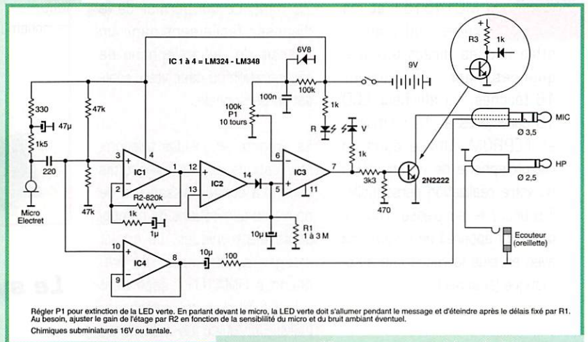
Vox pour portables/pédestre : Schéma valable pour Kenwood, pour autres marques voir notice de l'appareil.
