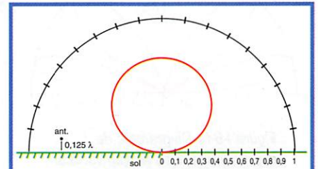
Figure 1-6-b : Diagramme de rayonnement dans le plan vertical d'un doublet demi-onde, fil horizontal placé à 0,123 \lambda du sol.
