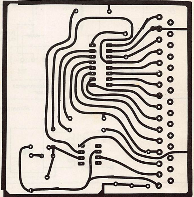
Circuit imprimé vu de dessus
