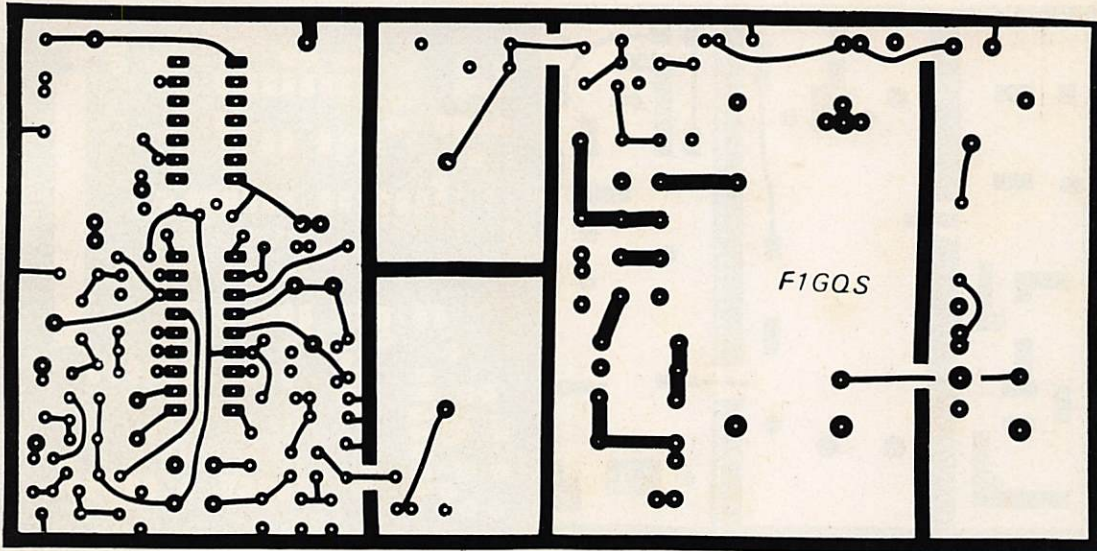
RECEPTION COTE SOUDURES
