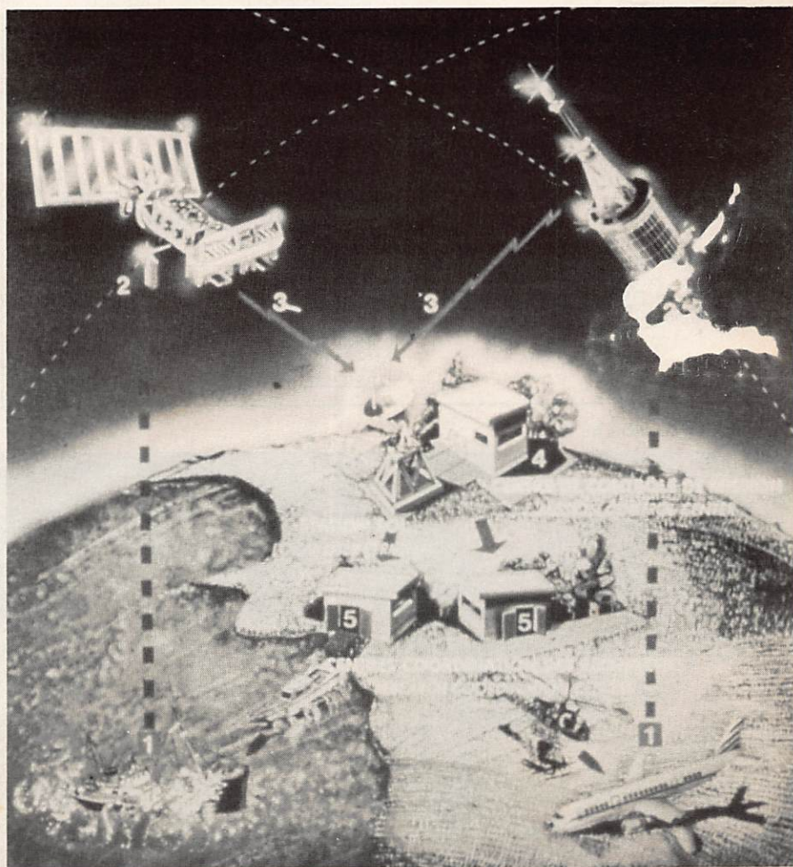
Principe du système SARTSAT-COSPAS
