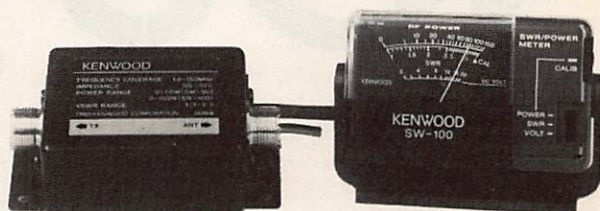
WATTMETRE / TOS - METRE SW 100 A - HF - VHF SW 100 B - VHF - UHF Sonde extérieure à l'appareil de mesure
