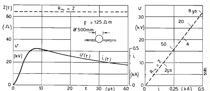
Fig. 1. — Dispersori di terra localizzati. Comportamento ad impulso, per piccoli valori di corrente impressa.
