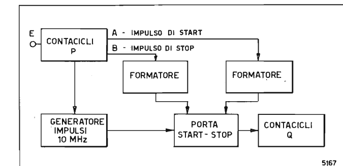
Fig. 8. — Schema a blocchi del sistema di misura impiegato per i rilievi sperimentali sui segnali di filodiffusione.
