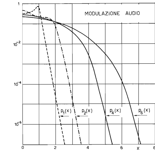
Fig. 11. — Andamento della funzione di densità di probabilità dei valori istantanei del segnale risultante da 1, 2, 4 e 6 portanti di ampiezza unitaria modulate dal segnale audio.
