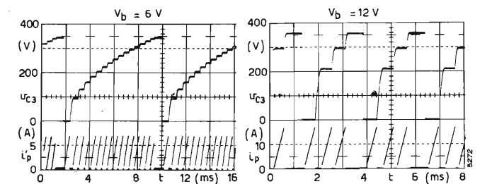
Fig. 9. — Andamento della tensione ai capi della capacità C_3 ( V_{C3} ) e della corrente nell'avvolgimento primario N_p' ( i_p ) in funzione del tempo t , per due diversi valori della tensione della batteria di alimentazione ( V_b ).
