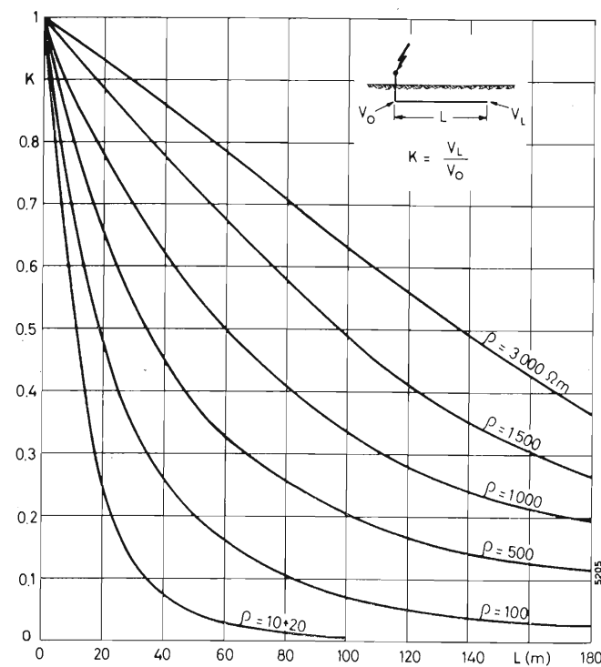
Fig. 10. — Andamento del rapporto tra i valori di cresta della tensione V_L all'estremità finale e V_0 alla estremità iniziale e di fili interrati di diversa lunghezza L .
