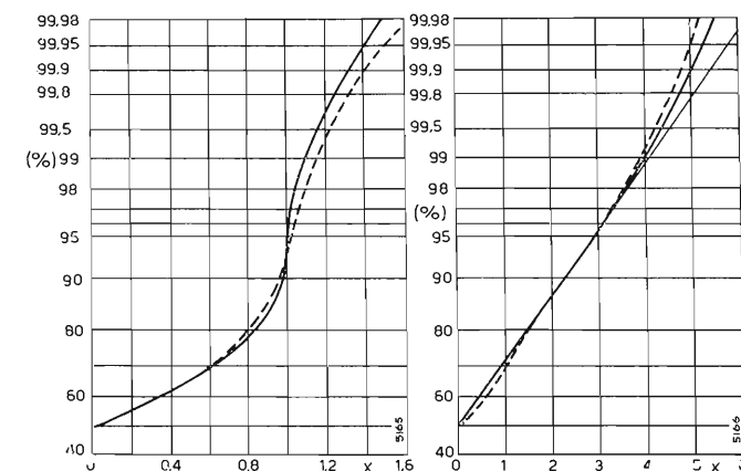
Fig. 6. — Distribuzione di probabilità di una portante di ampiezza unitaria modulata dal segnale vocale; a tratti la curva sperimentale ricavata su un singolo canale di filodiffusione.
