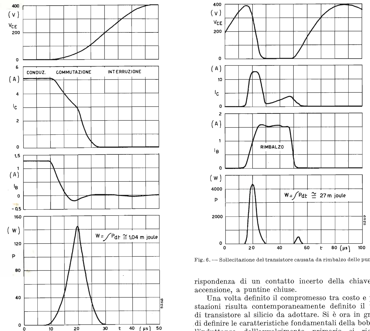
Fig. 5. — Sollecitazioni a cui è sottoposto il transistor finale durante commutazione.
