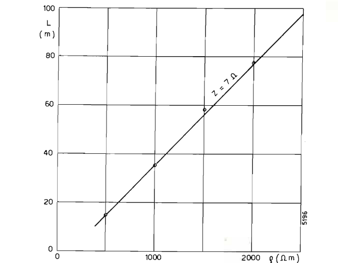
Fig. 16. — Protezione dalle tensioni di passo: dimensioni minime del dispersore.
