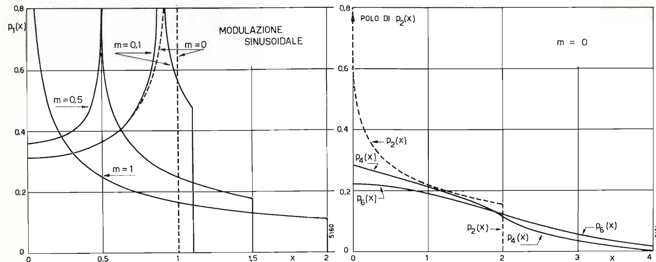
Fig. 1. — Densità di probabilità di una sinusoide di ampiezza unitaria modulata da una sinusoide con vari valori della profondità di modulazione m .
