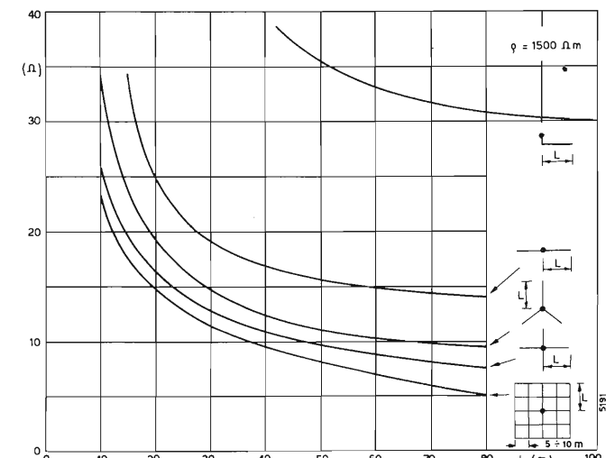
Fig. 11. — Impedenza ad impulso di stelle ad n raggi al variare della loro lunghezza L .
