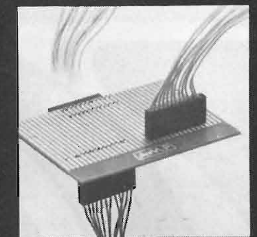
Connessione scheda-filo
