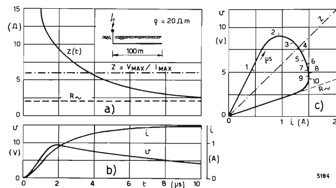
Fig. 4. — Dispersioni di terra estesi. Comportamento ad impulso, per piccoli valori di corrente impressa.
