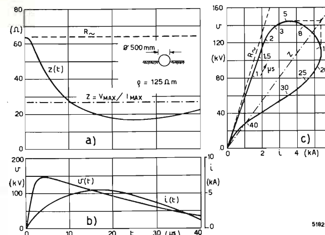
Fig. 2. — Dispersori di terra localizzati. Comportamento da impulso, per grandi valori di corrente impressa.
