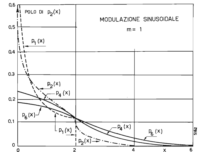
Fig. 3. — Densità di probabilità dei valori istantanei di un segnale di somma di 1, 2, 4 e 6 sinusoidi modulate sinusoidalmente al 100% ( m = 1 ).
