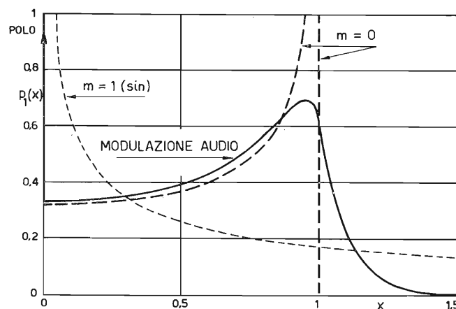
Fig. 10. — Andamento della p_1(x) ; con linea continua: portante di ampiezza unitaria modulata dal segnale audio; a tratti: sinusoide non modulata ( m = 0 ); punteggiata: portante modulata sinusoidalmente al 100% ( m = 1 ).
