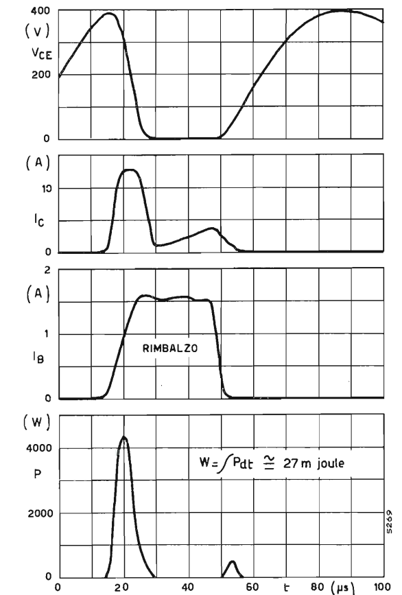
Fig. 6. — Sollecitazione del transistor causata da rimbalzo delle puntine.
