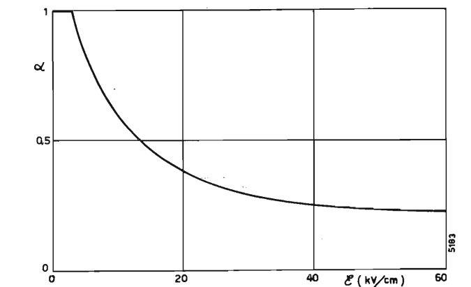
Fig. 3. — Dispersori di terra localizzati. Dipendenza dell'efficienza ad impulso dell'intensità del campo elettrico.
