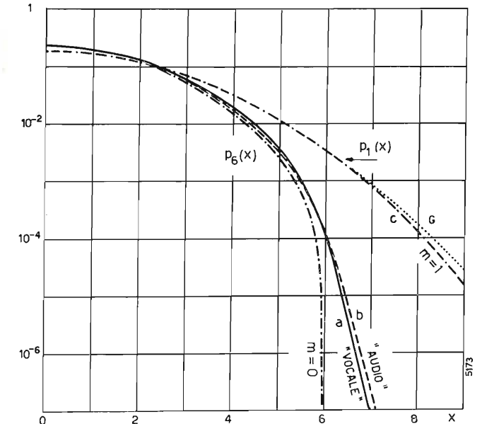
Fig. 14. — Densità di probabilità del segnale somma di 6 portanti di ampiezza unitaria modulate da segnali di differenti proprietà statistiche. Con G è indicata la gaussiana avente lo stesso scarto quadratico medio della curva relativa al segnale somma di 6 portanti modulate sinusoidalmente al 100%.
