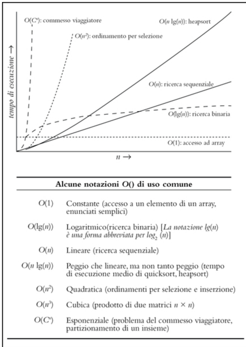
Figura 6.1 Tempi di esecuzione di vari algoritmi.
