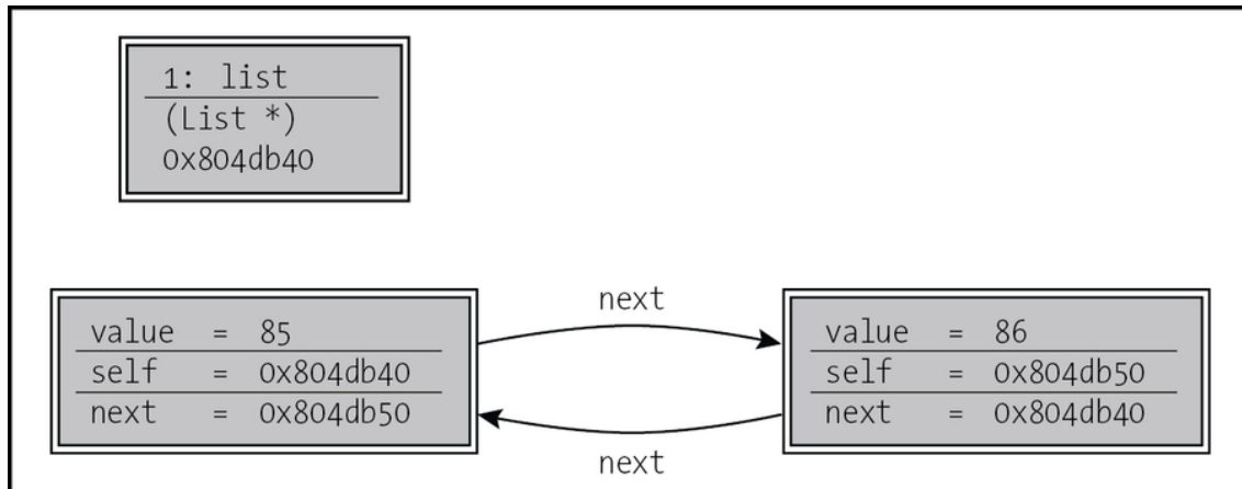
Figura 3.2 Esempio di diagramma da debugger di una lista concatenata circolare. Le frecce rappresentano puntatori a nodi.
